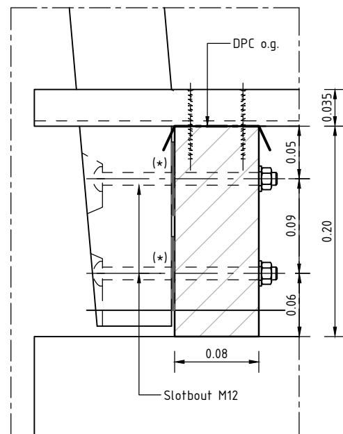
Detail 1 schaal 1:5
