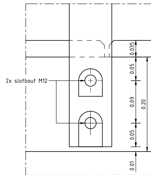
Detail 3 schaal 1:5
