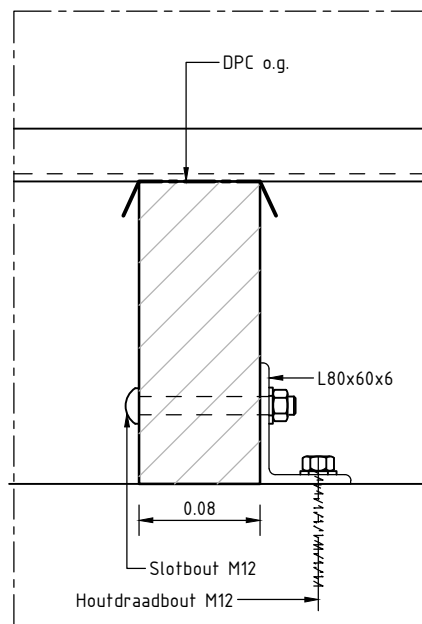
Detail 2 schaal 1:5
