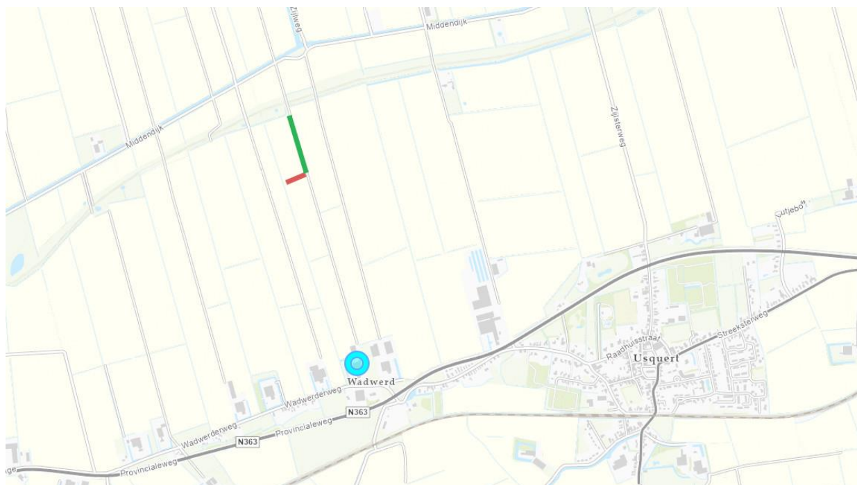
Figuur 1: Locatie van werkzaamheden. De rode lijn geeft te dempen watergang weer. De groene lijn geeft te verbreden watergang weer.
