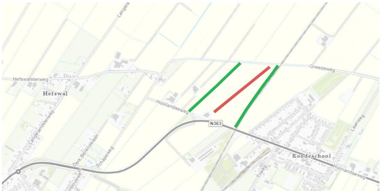
Figuur 1: Locatie van werkzaamheden. De rode lijnen geven te dempen watergangen weer. De groen lijnen geven te verbreden watergangen weer.
