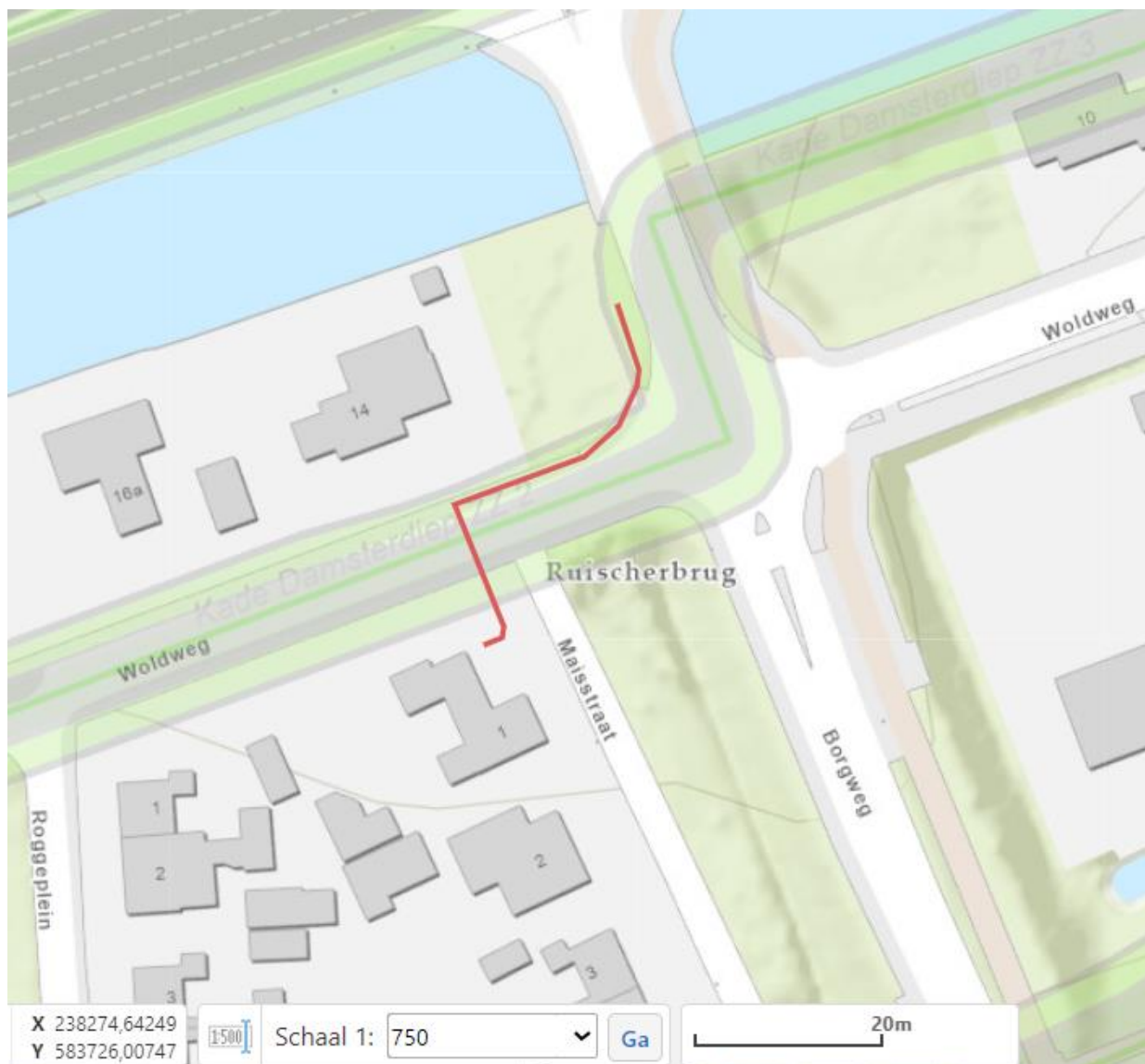
Figuur 2: Schematische tekening van de werkzaamheden. De rode lijn geeft globaal de locatie weer van de aan te leggen waterleiding.
