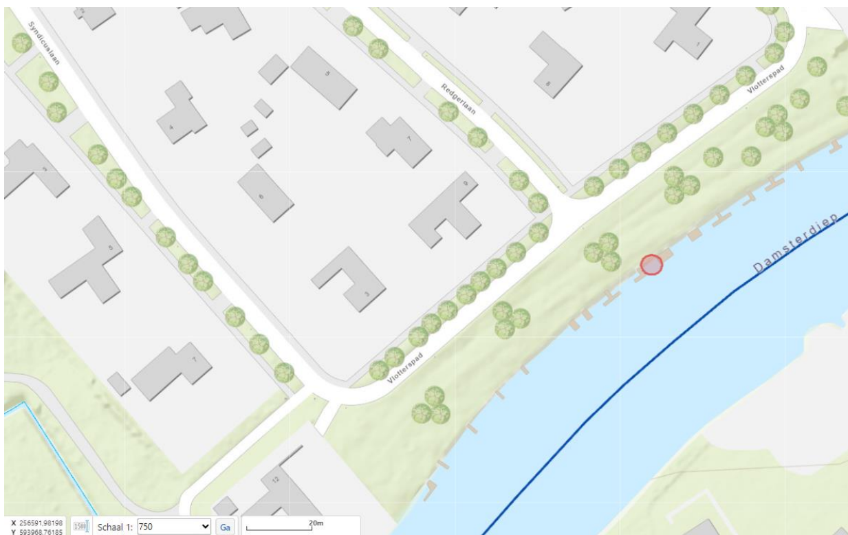
Figuur 1: Schematische tekening van de werkzaamheden. De rode cirkel geeft globaal de locatie weer van de aan te leggen steiger.
