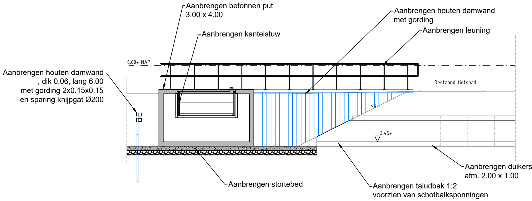
PRINCIPE PROFIEL A Schaal 1:100
