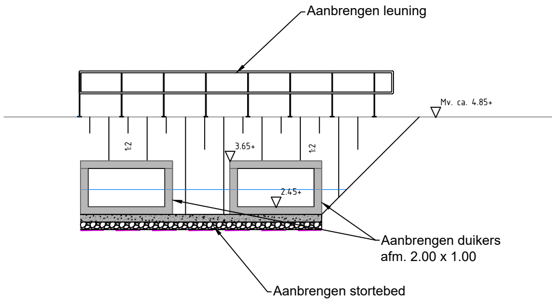
PRINCIPE PROFIEL B Schaal 1:100
