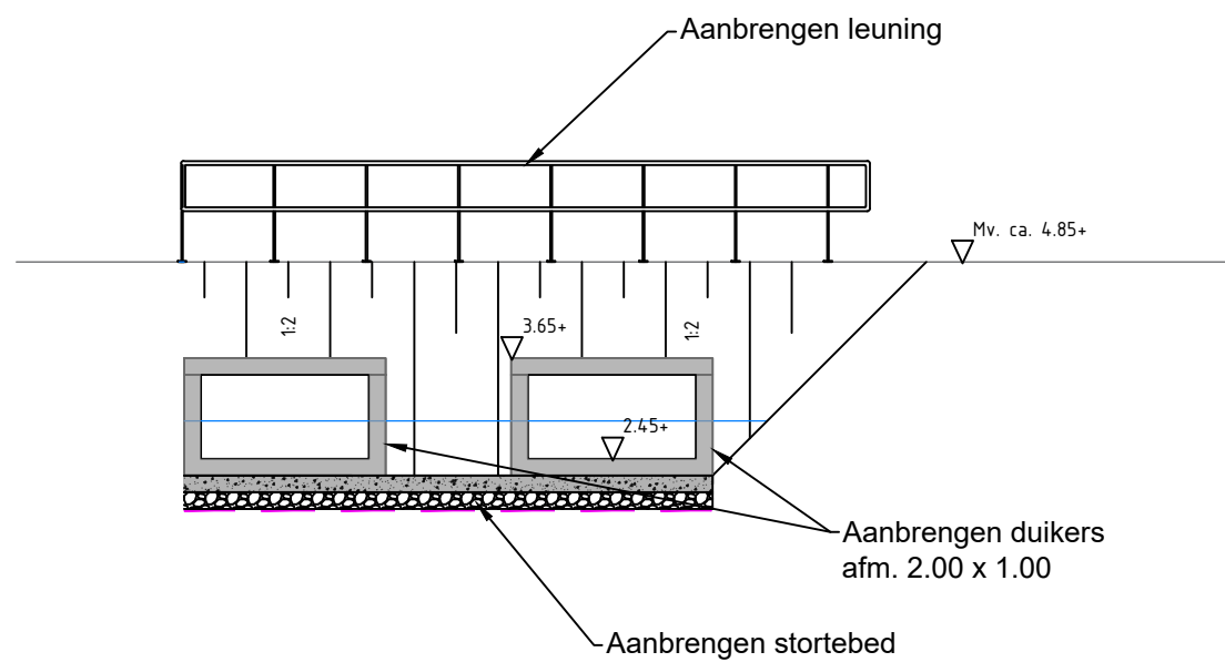
PRINCIPE PROFIEL B Schaal 1:100
