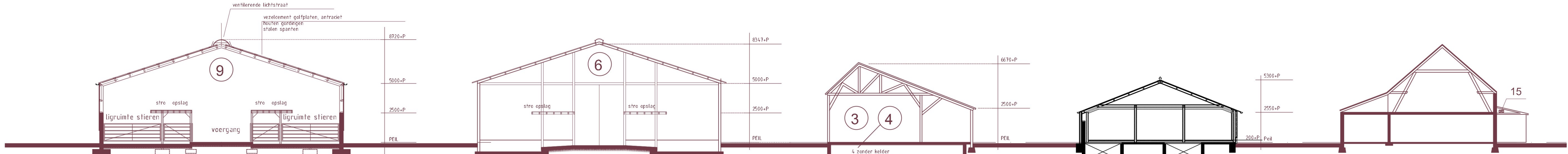
DOORSNEDE GEBOUW 9
