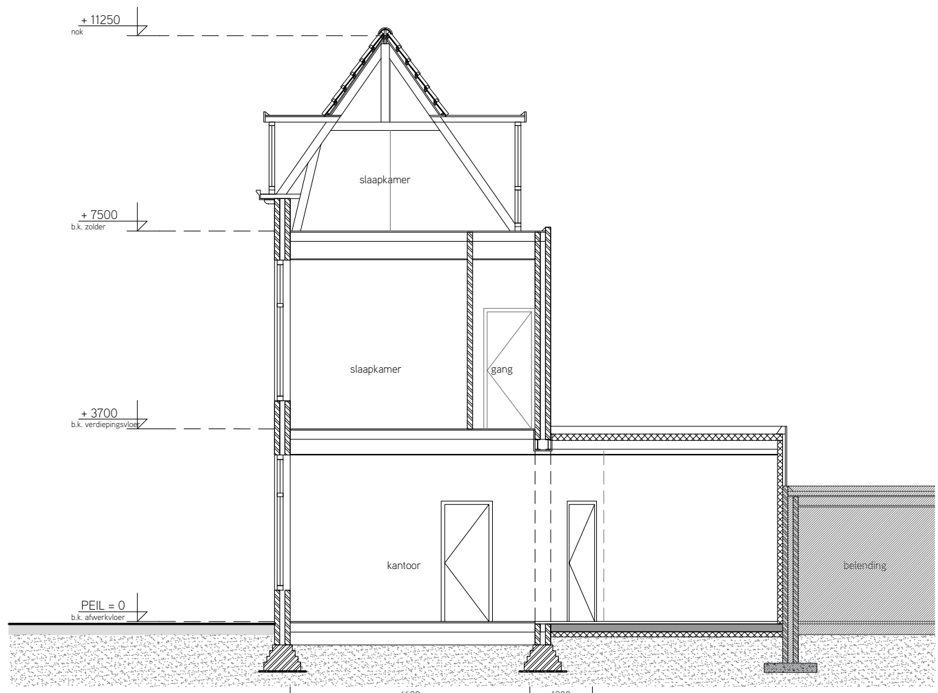
Doorsnede AA bekend archief
