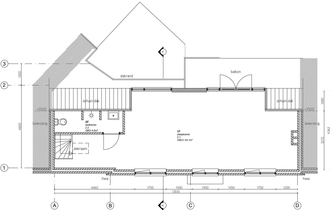
Zolder verdieping bekend archief +7500
