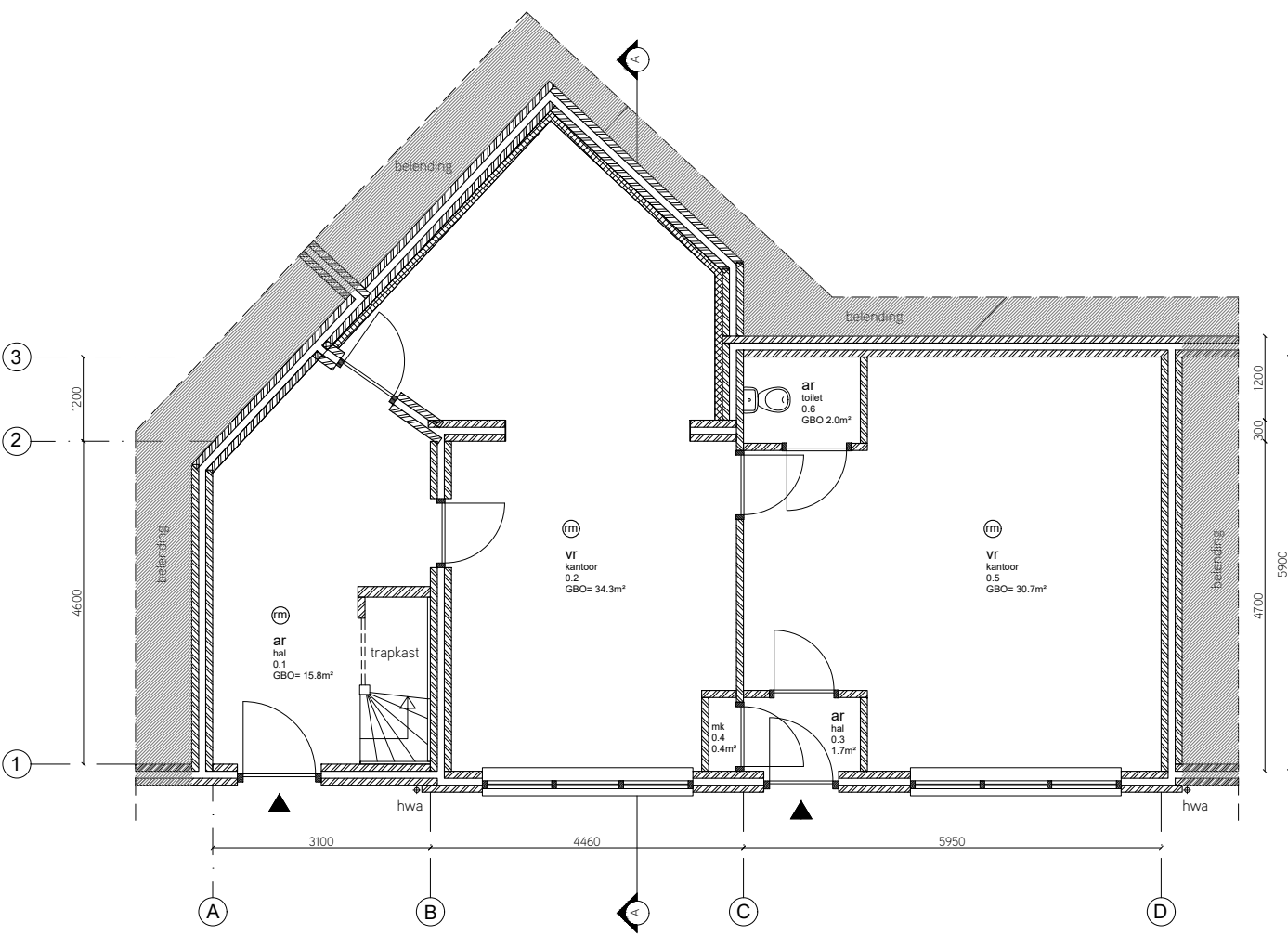
Begane grond bekend archief +0
