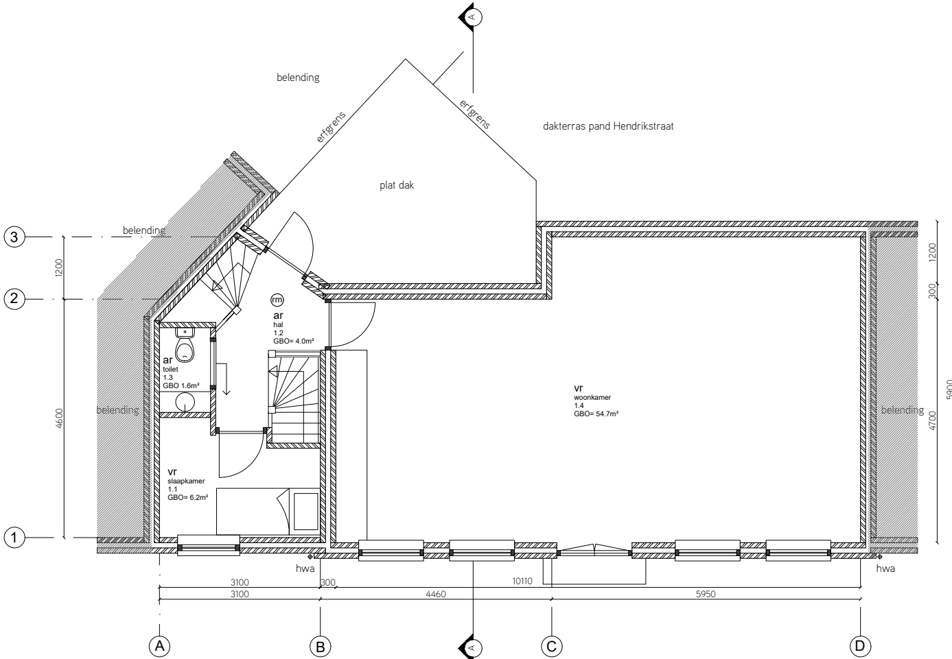
Eerste verdieping feitelijke situatie +3700
