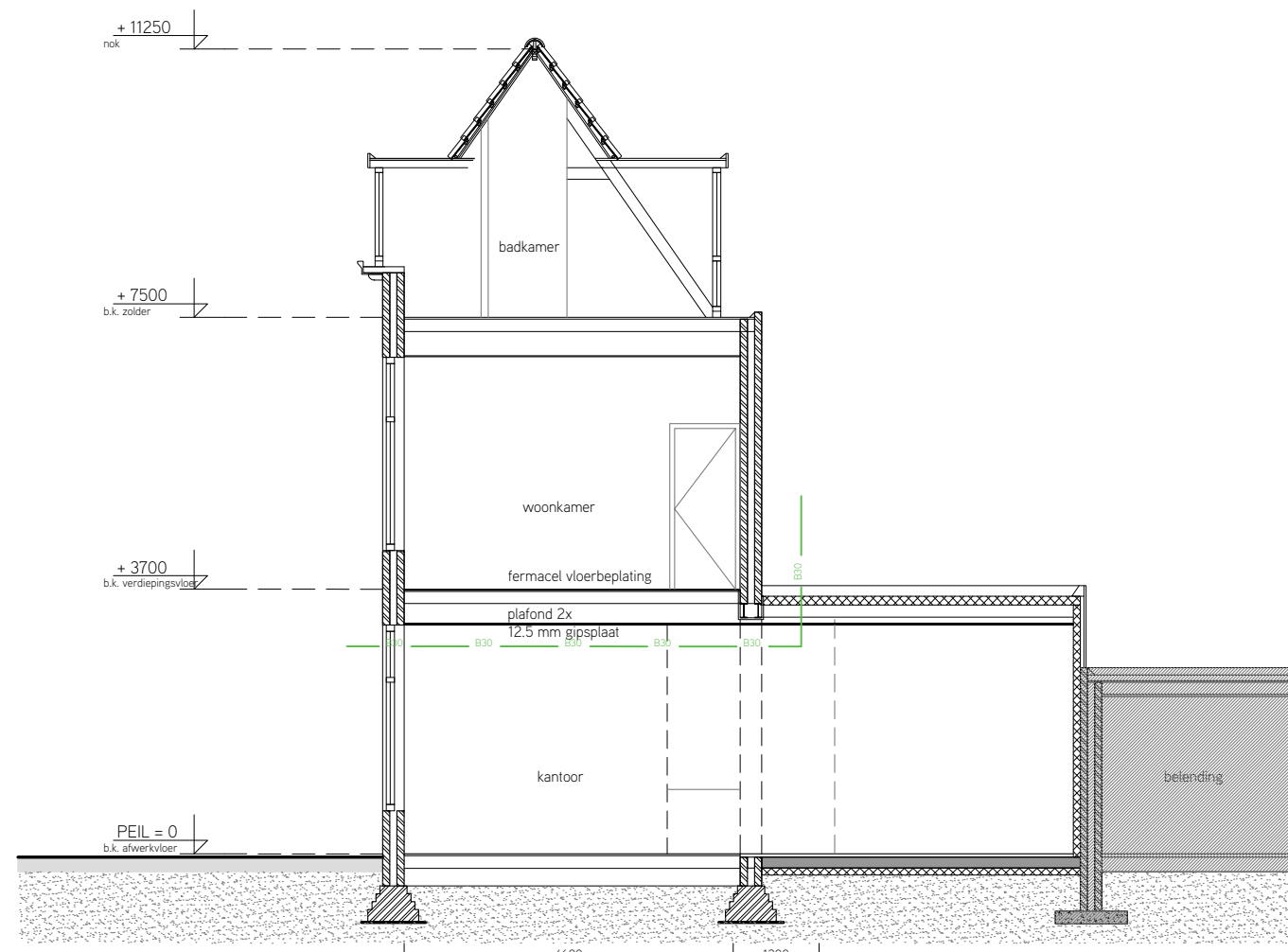
Doorsnede AA feitelijke situatie
