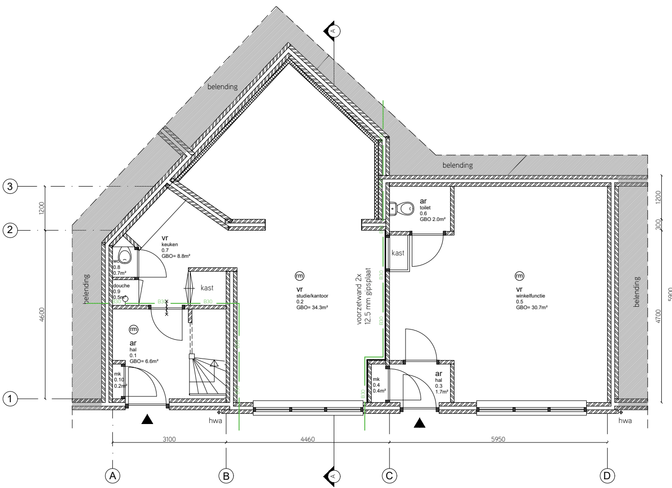
Begane grond feitelijke situatie +0
