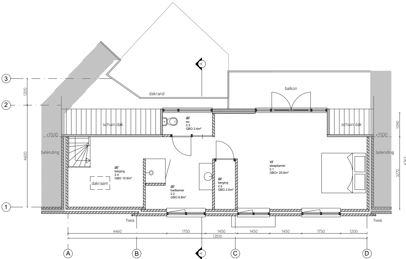
Zolder verdieping feitelijke situatie +7500
