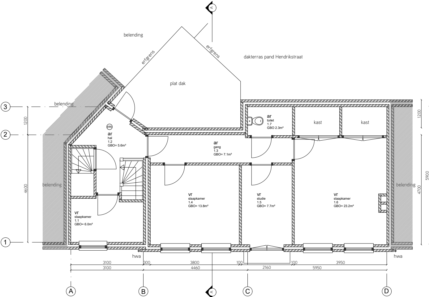
Eerste verdieping bekend archief +3700
