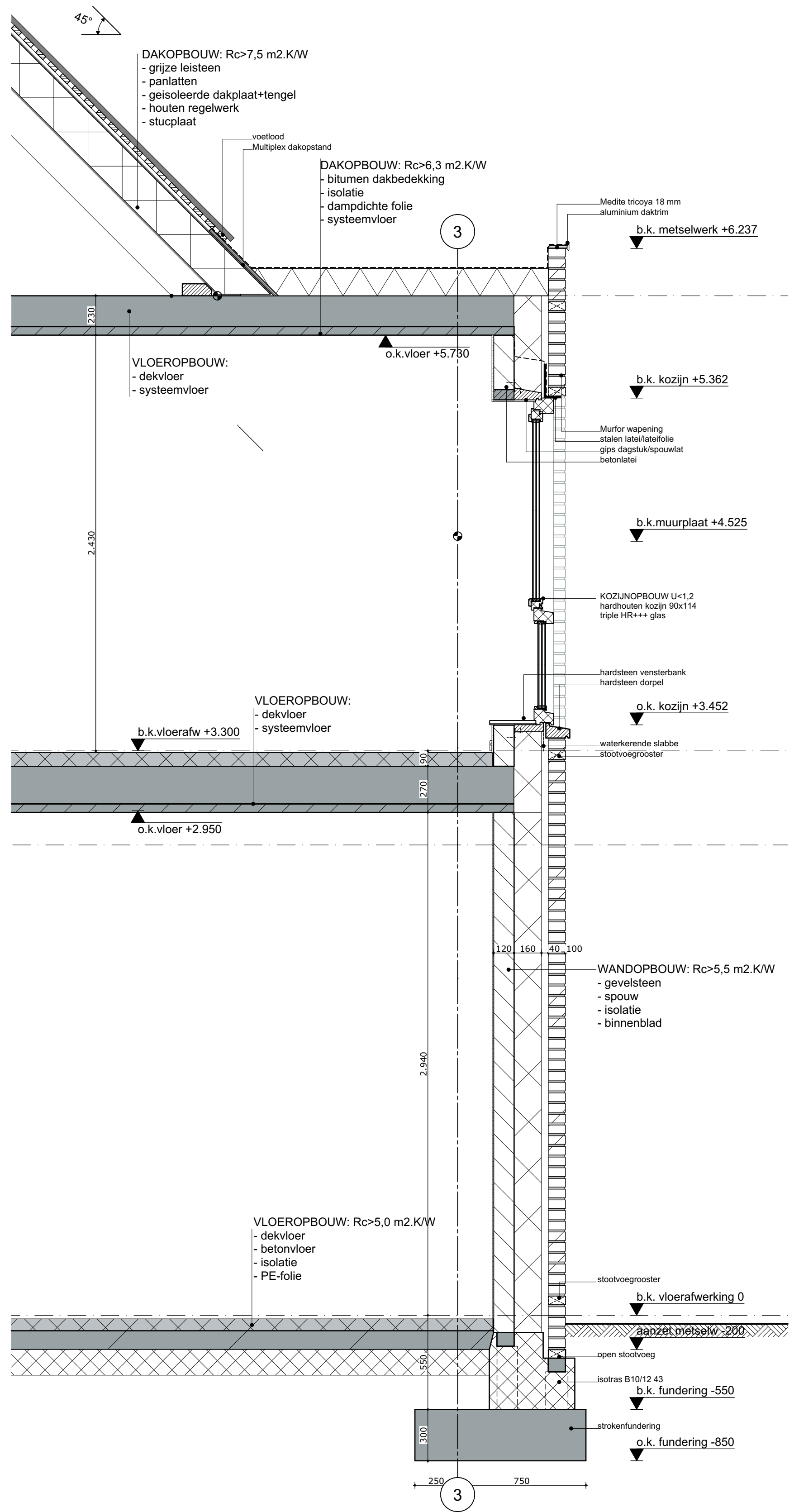
DETAILDOORSNEDE 03
