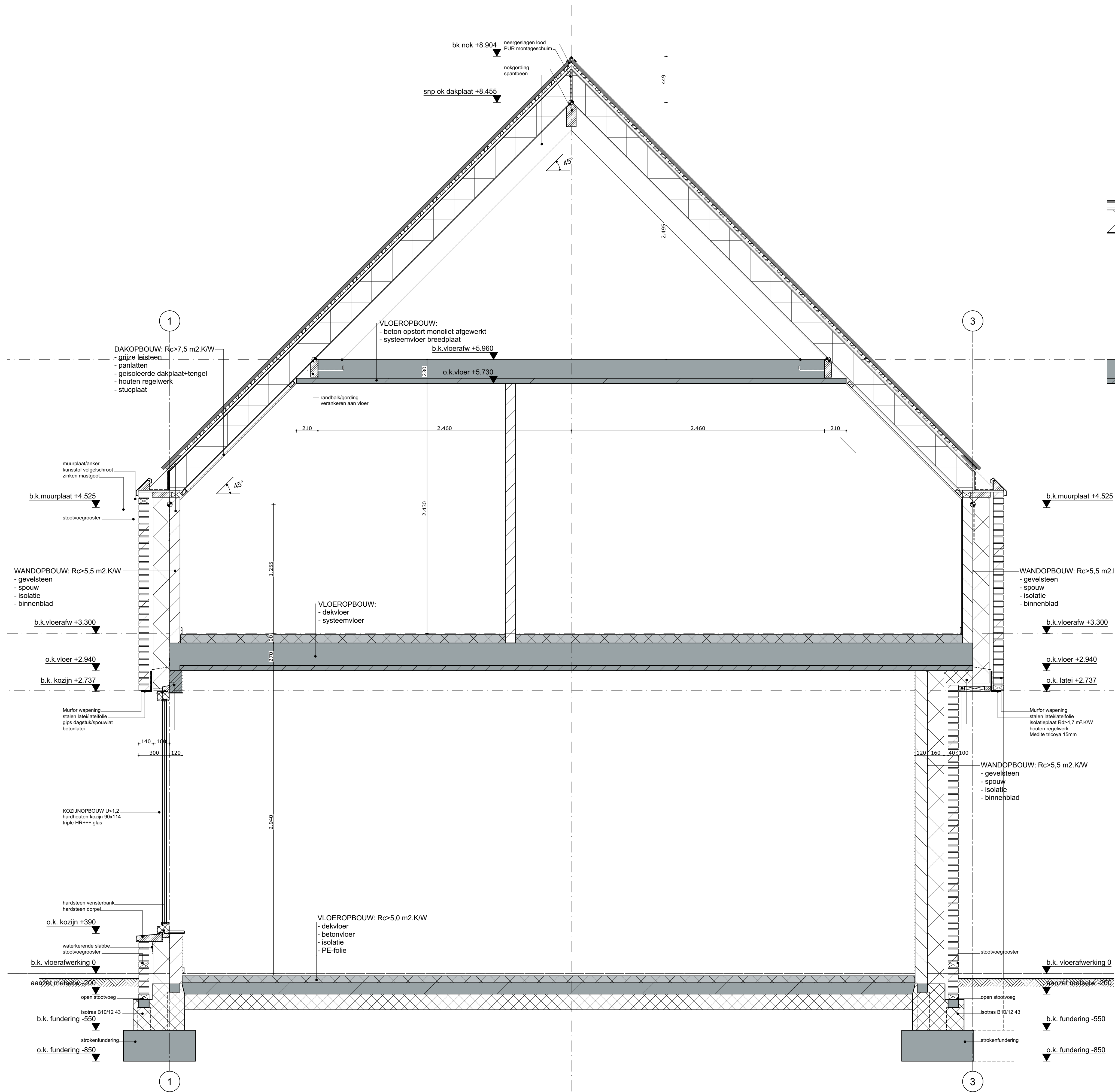
DETAILDOORSNEDE 01
