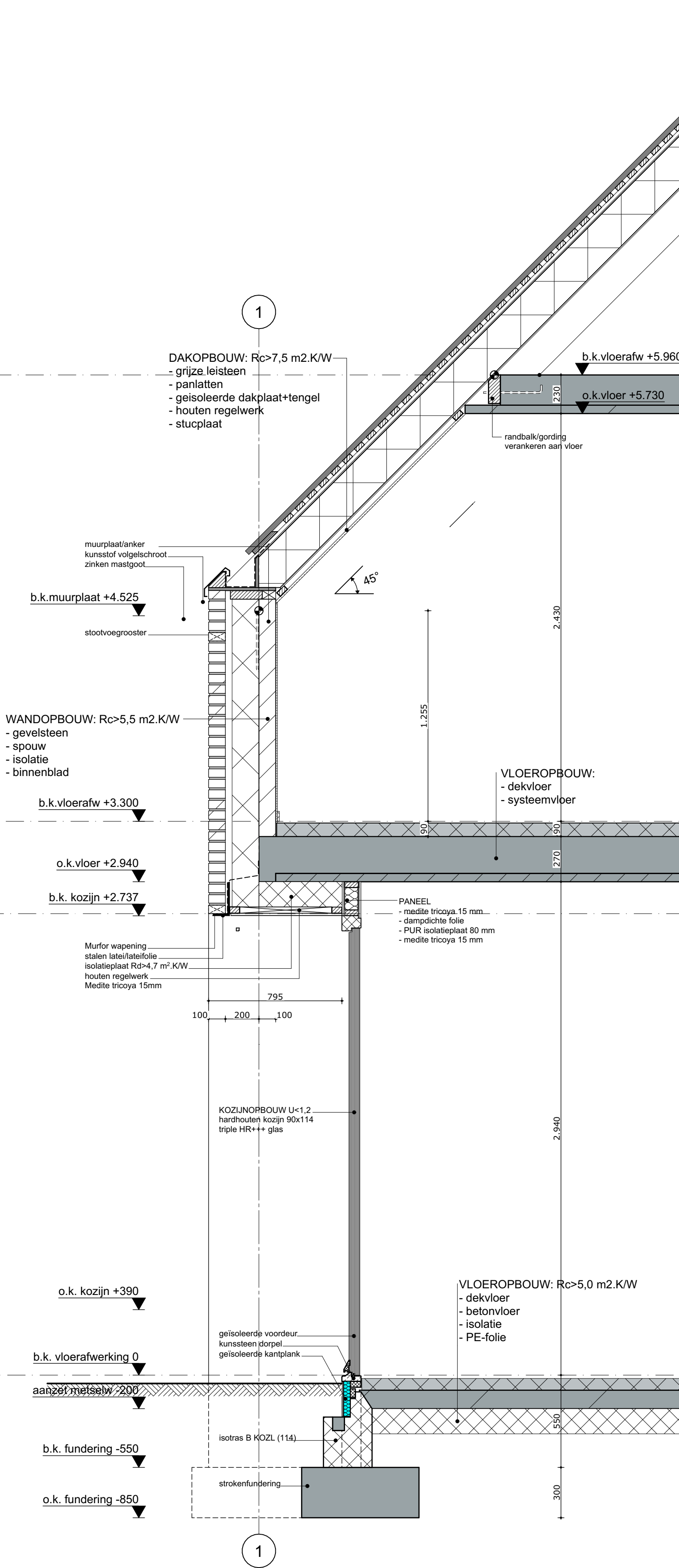
DETAILDOORSNEDE 02
