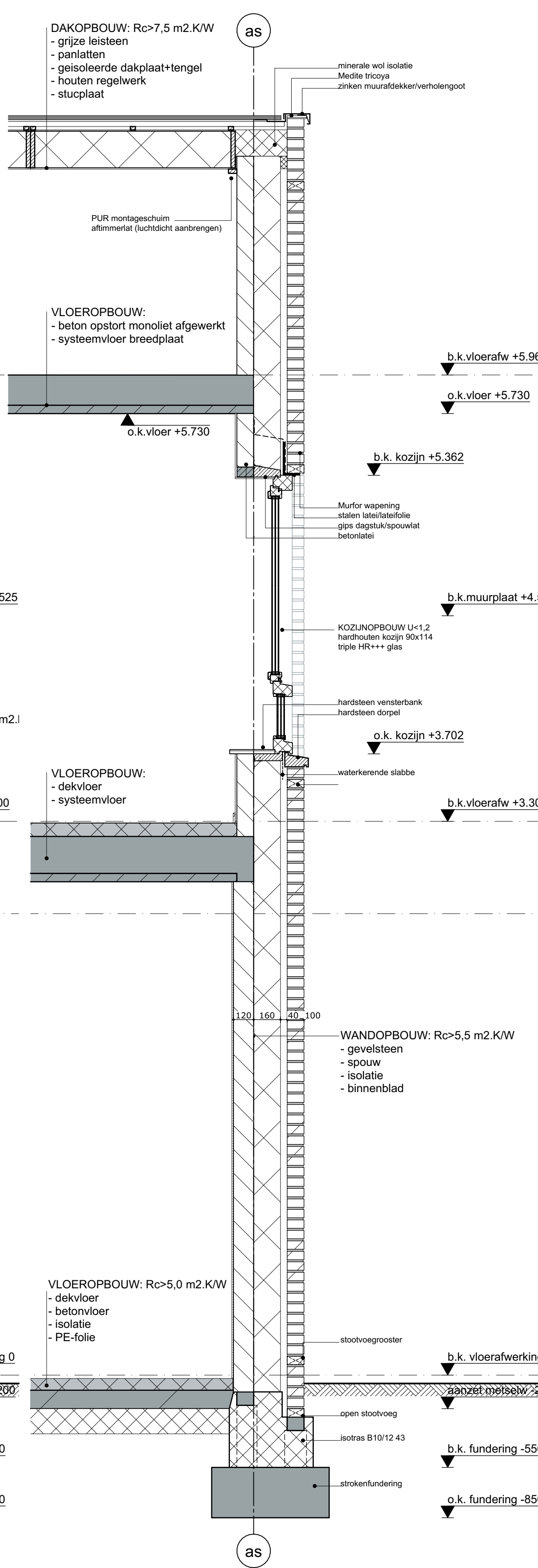
DETAILDOORSNEDE 04
