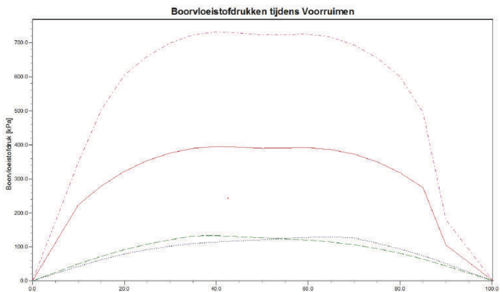
Figuur 9 Boorvloeistof tijdens Ruim- en intrekoperatie
