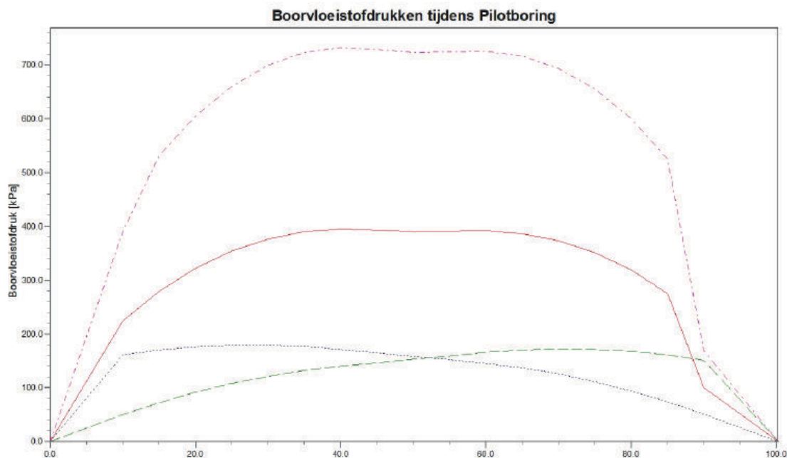
Figuur 7 Boorvloeistof tijdens Pilotboring
