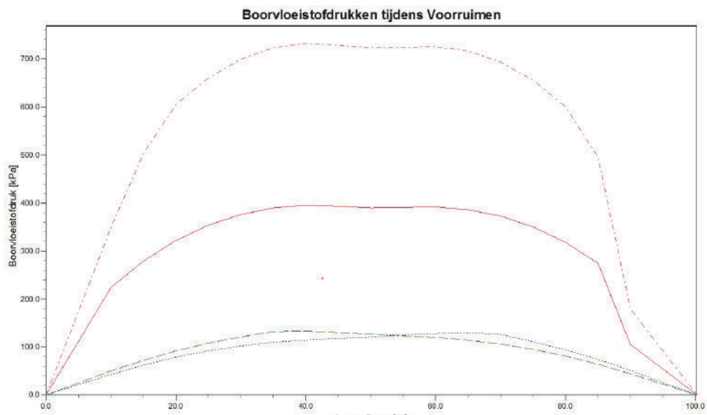
Figuur 8 Boorvloeistof tijdens Voorruimen
