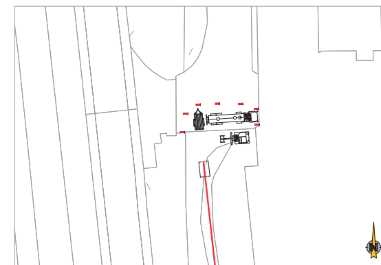
INDICATIEVE OPSTELLING ITP SCHAAL M 1:200
