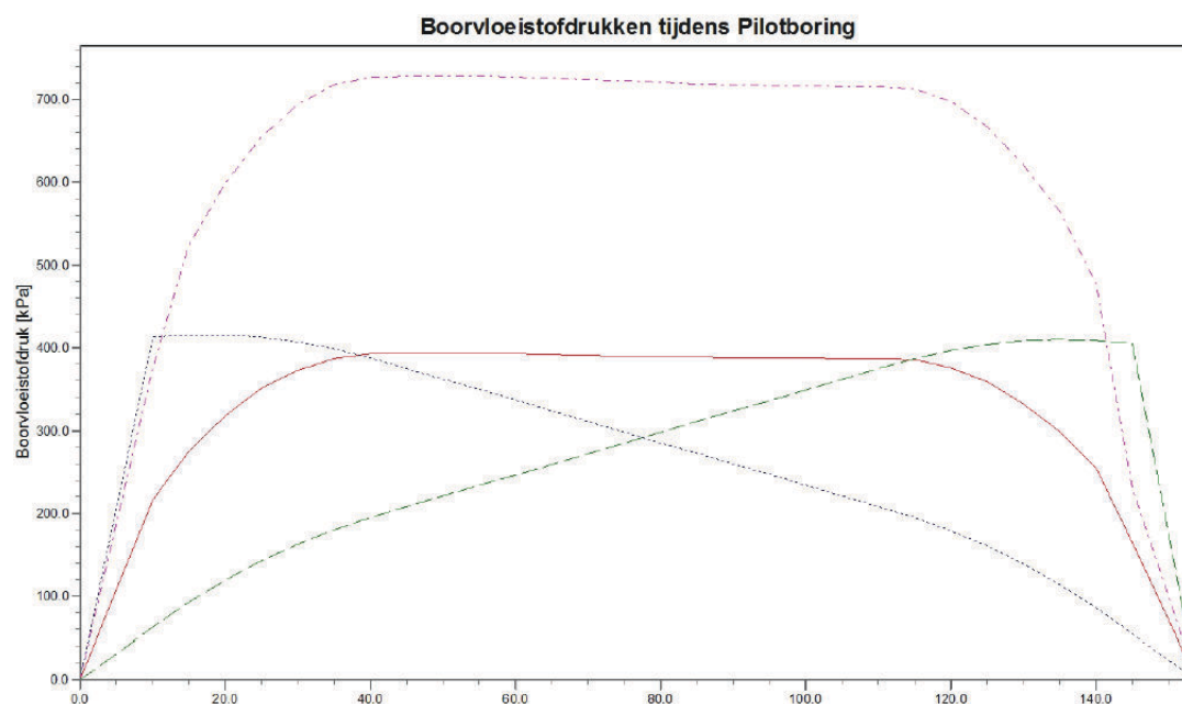
Figuur 7 Boorvloeistof tijdens Pilotboring
