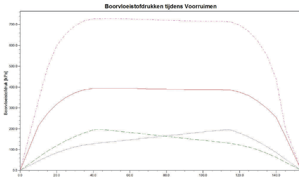
Figuur 9 Boorvloeistof tijdens Ruim- en intrekooperatie
