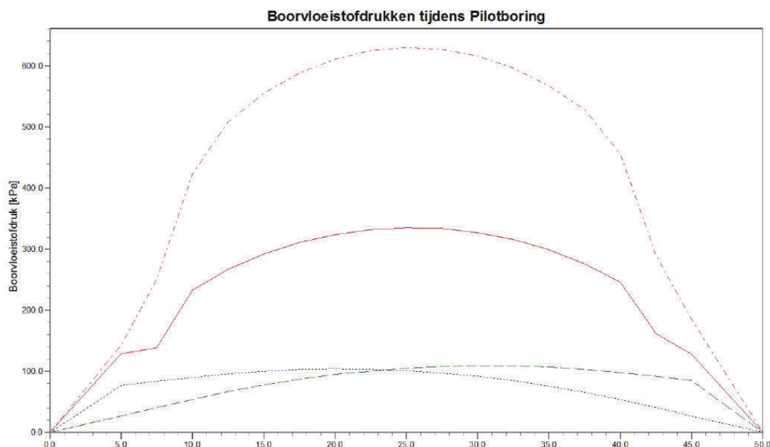
Figuur 7 Boorvloeistof tijdens Pilotboring
