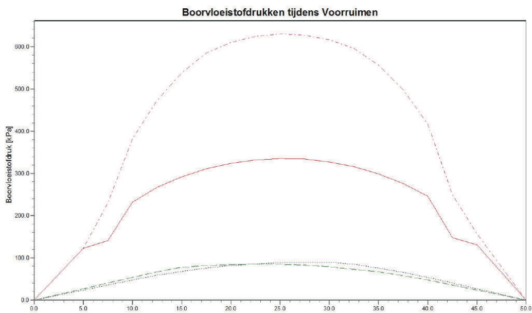
Figuur 9 Boorvloeistof tijdens Ruim- en intrekkoperatie
