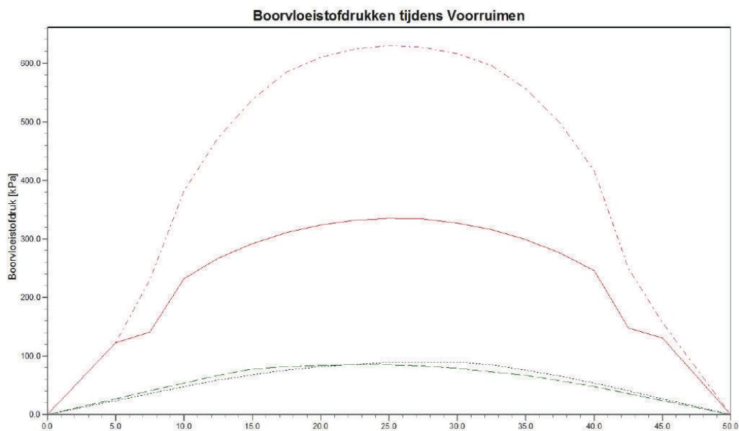
Figuur 8 Boorvloeistof tijdens Voorruimen
