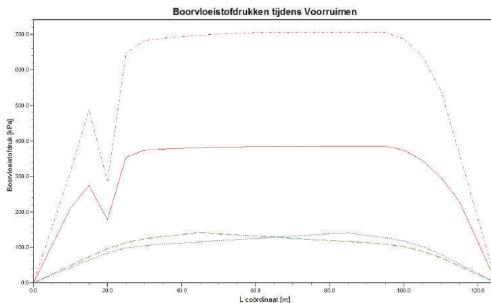
Figuur 9 Boorvloeistof tijdens Ruim- en intrekoperatie
