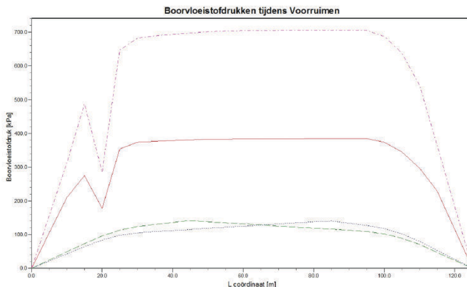
Figuur 8 Boorvloeistof tijdens Voorruimen
