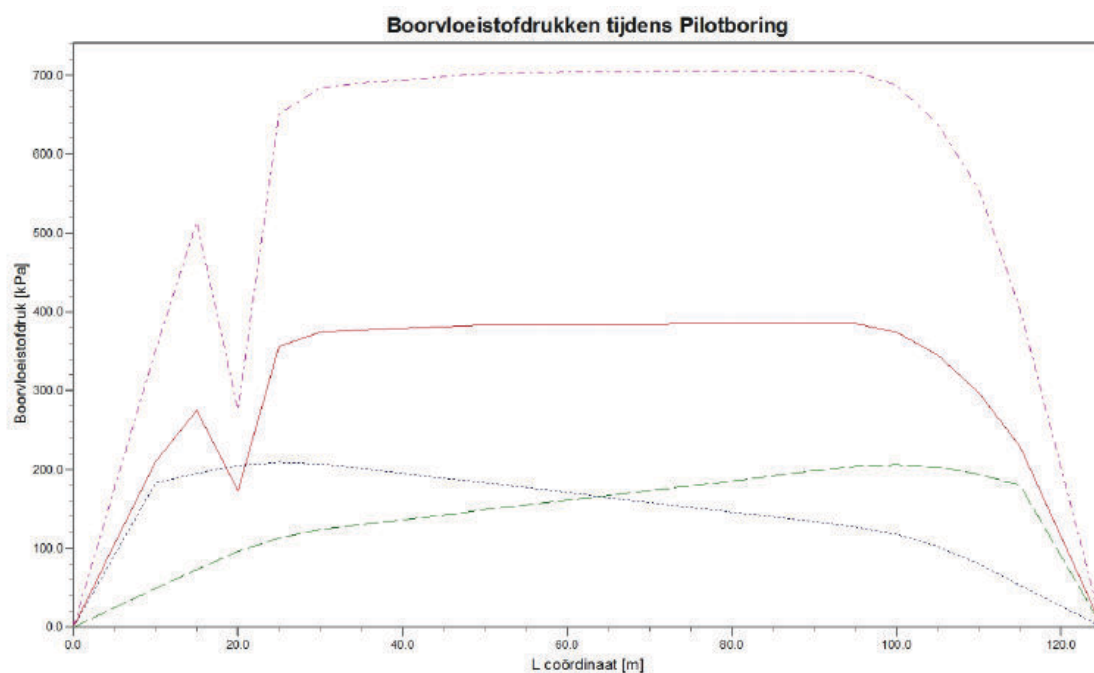
Figuur 7 Boorvloeistof tijdens Pilotboring
