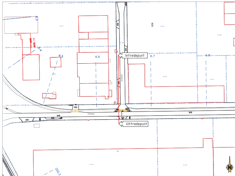
OVERZICHT SCHAL M_1:1000
