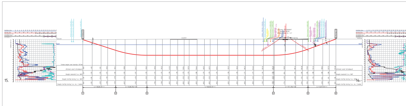
DWARSPROFIEL SCHAL Custom
