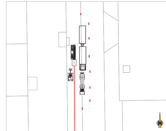
INDICATIEVE OPSTELLING ITP SCHAL M_1:200
