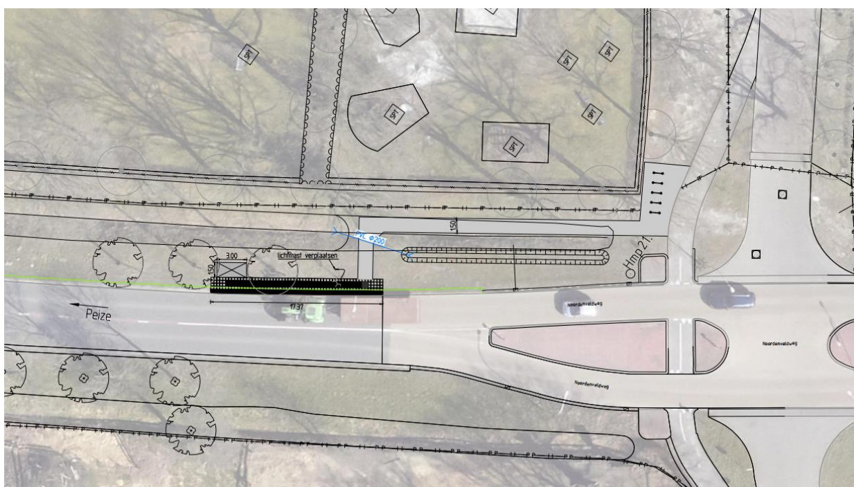
Figuur 1: Bovenaanzicht dam met duiker in een secundaire watergang en het gedeeltelijk dempen van een secundaire watergang ter hoogte van kruispunt Noordenveldweg (N386) met de Oosterstraat/Dorpsweg te Donderen
