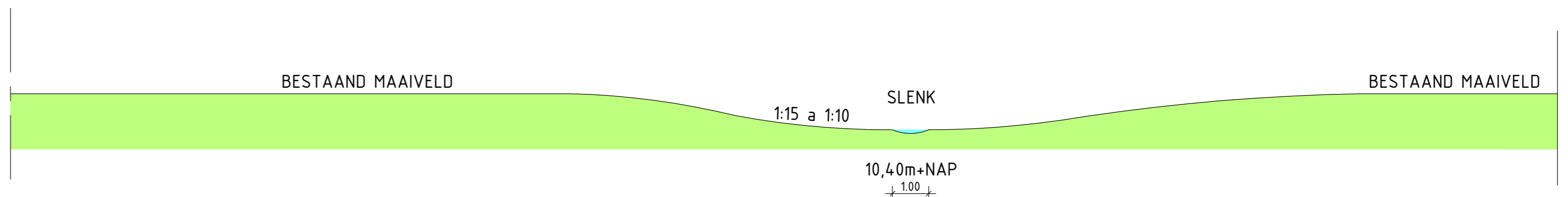
Schematische weergave DWP Slenk schaal 1:100
