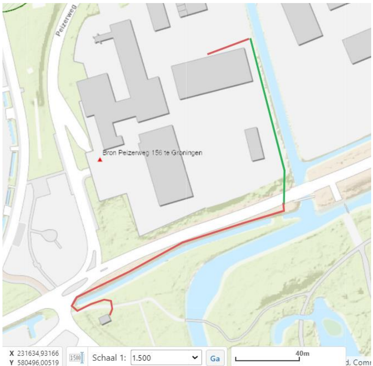
Figuur 1: Schematische tekening van de werkzaamheden. De rode lijn geeft globaal de locatie weer van de aan te leggen laagspanningskabels, het groene gedeelte geeft globaal de locatie weer van de gestuurde boring.
