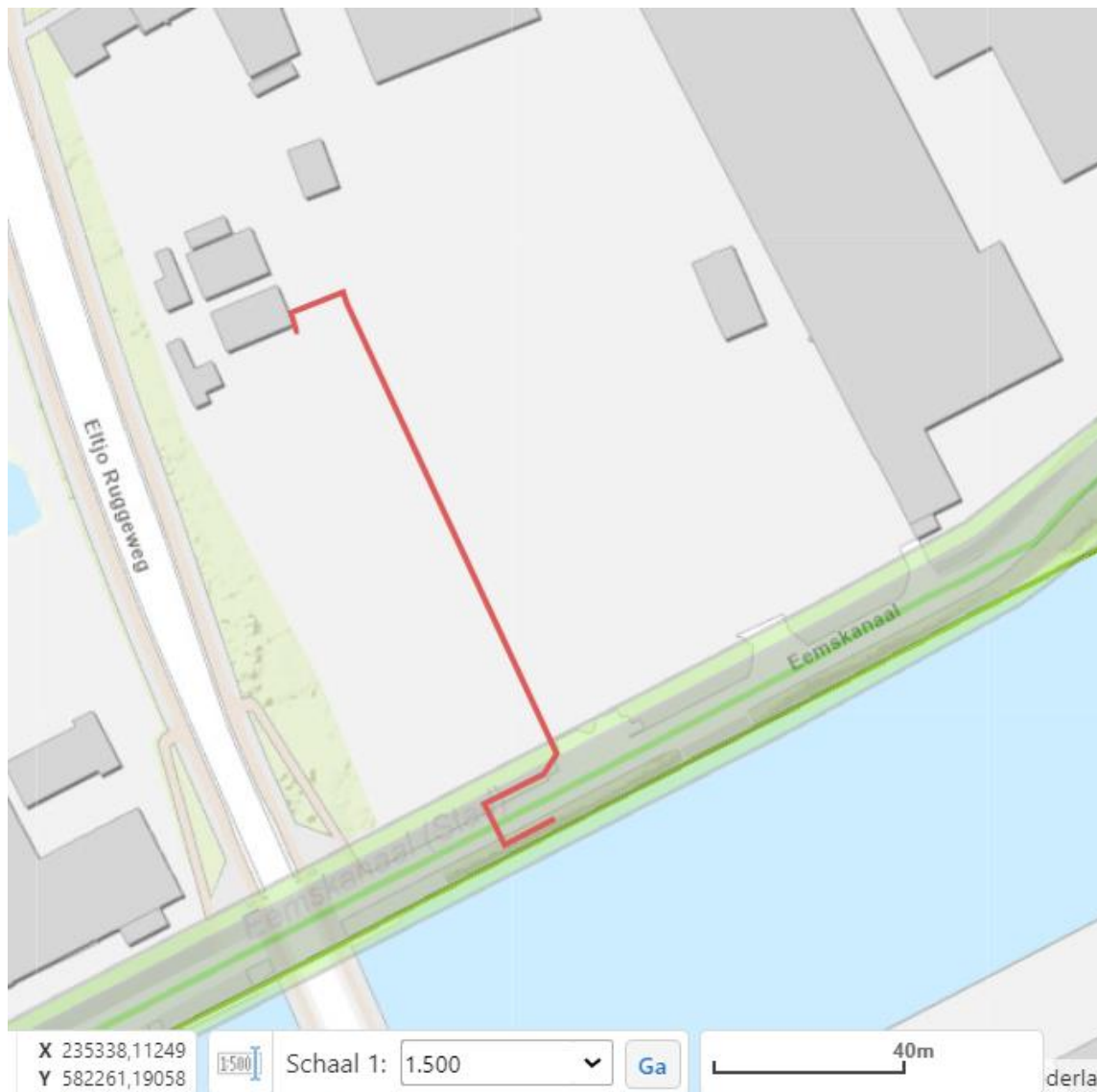
Figuur 1: Schematische tekening van de werkzaamheden. De rode lijn geeft globaal de locatie weer van de aan te leggen COAX kabel. Aan de zuidkant van het tracé bevindt zich de locatie van de te plaatsen straatkast.
