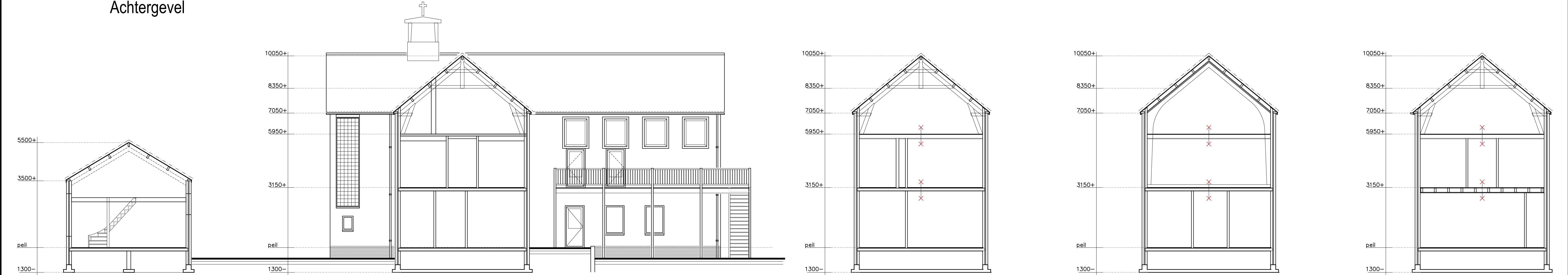
Doorsnede A
