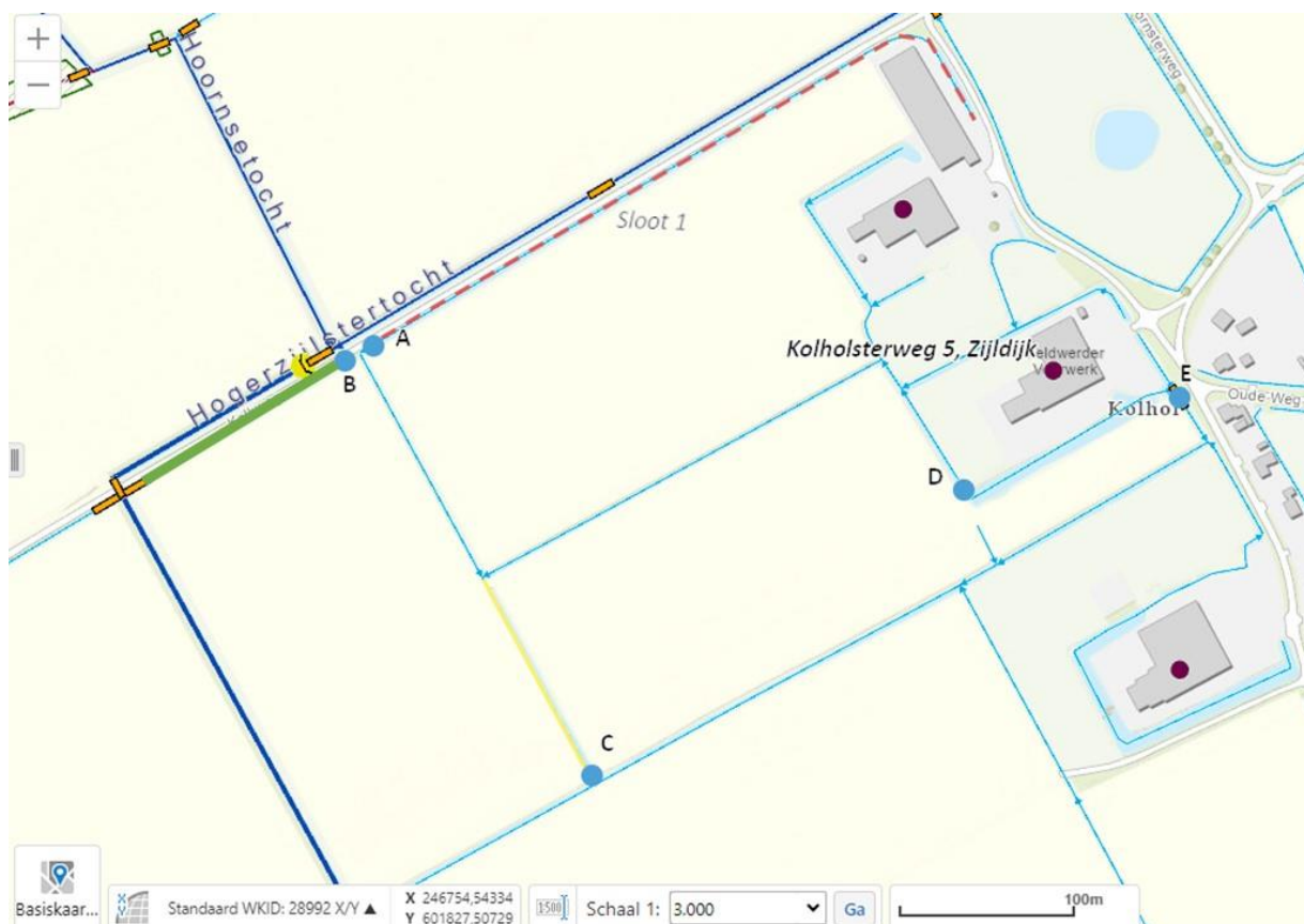
Figuur 1: Bovenaanzicht waterhuishoudkundige situatie met daarop aangegeven dam met duiker (punt A), te vervangen dam met duiker (punt B), te verwijderen duiker (punt C), te dempen watergang (gele streep) en de te verbreden watergang (doorgetrokken groene streep) ter hoogte van Kolholsterweg 5 te Zijldijk.
