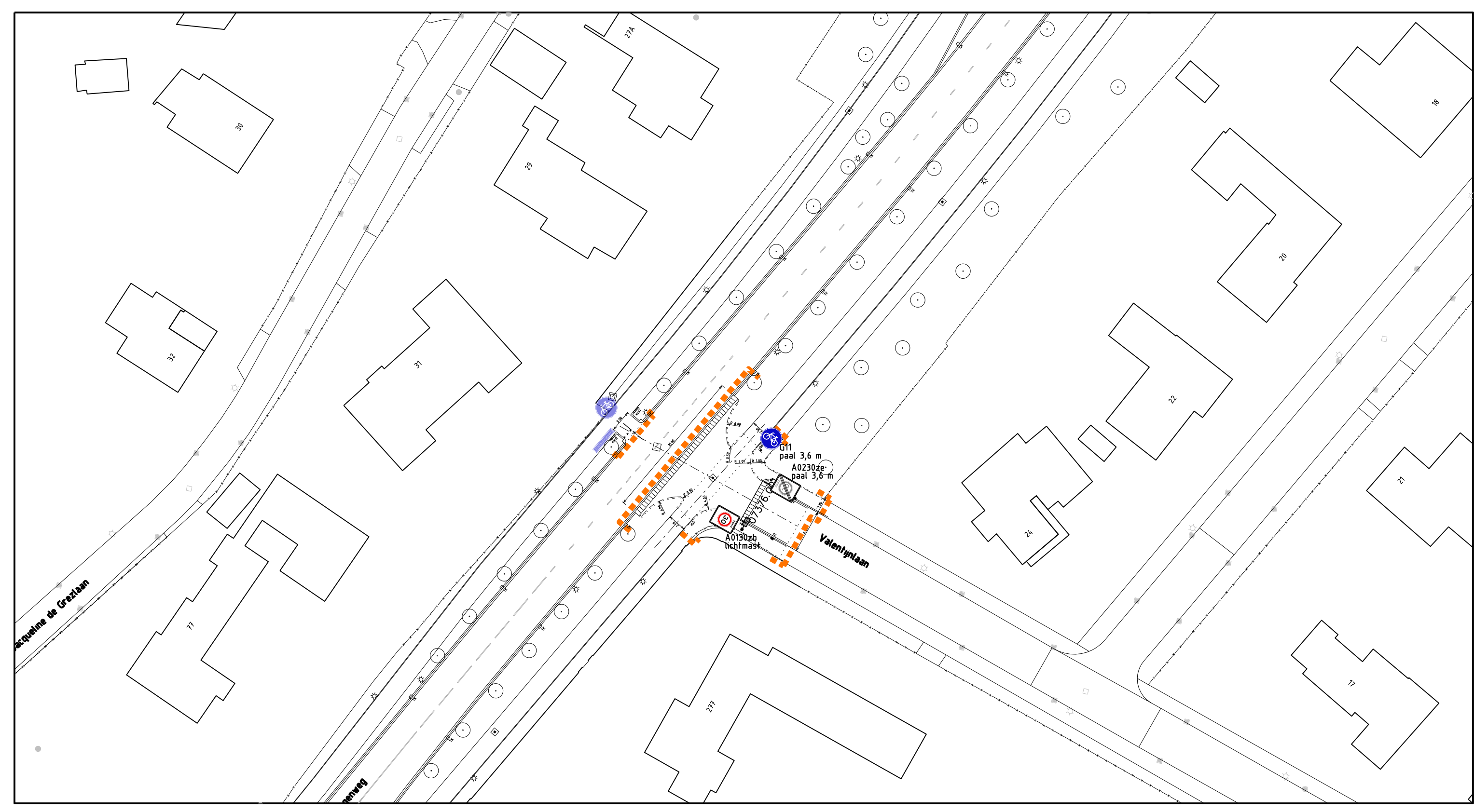
Overzicht: wijzigingen Valentijnlaan schaal 1:200
