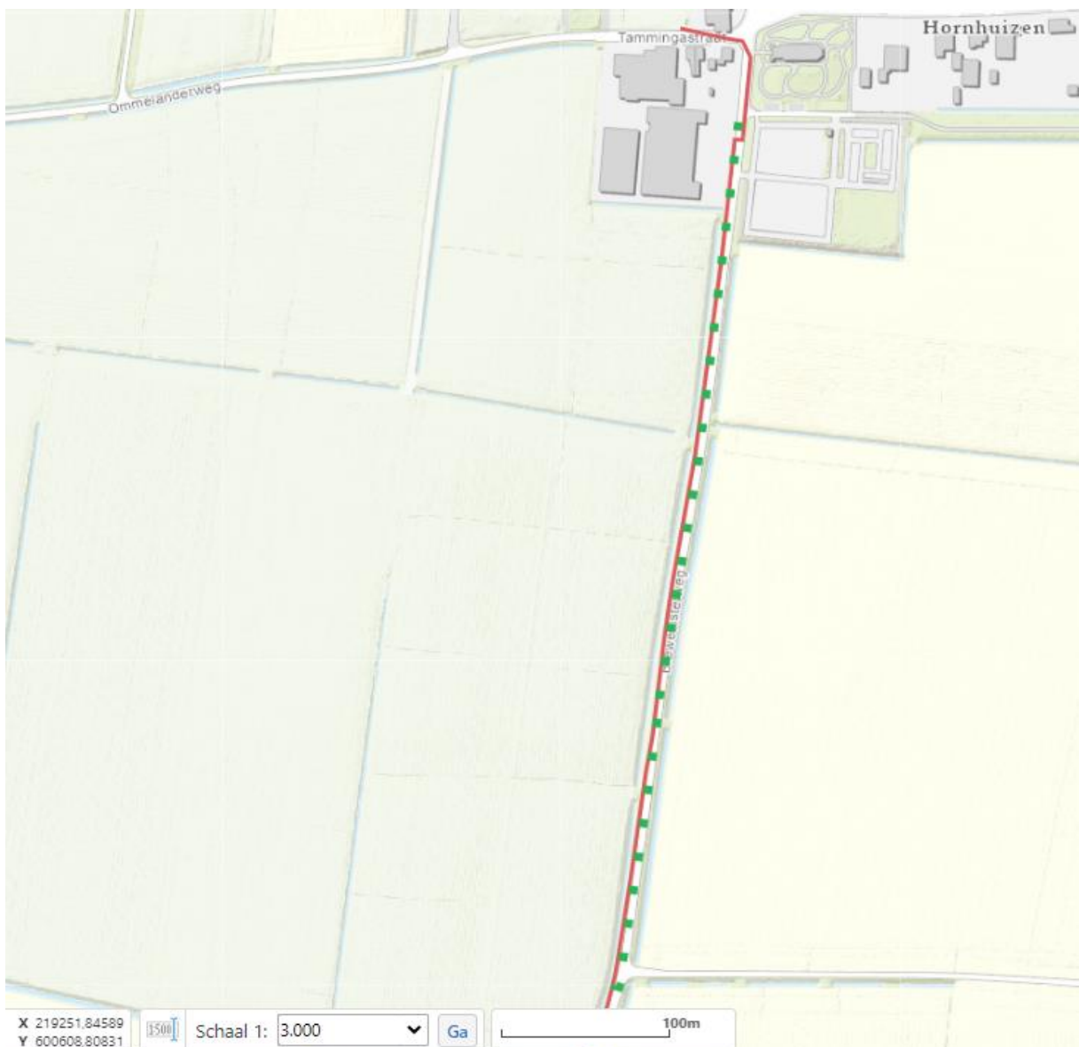
Figuur 1: Schematische tekening van de werkzaamheden. De rode lijn geeft globaal het aan te leggen tracé voor de middenspanningskabels weer en de groene stippellijn geeft globaal de locatie weer van de aan te leggen gasleiding.
