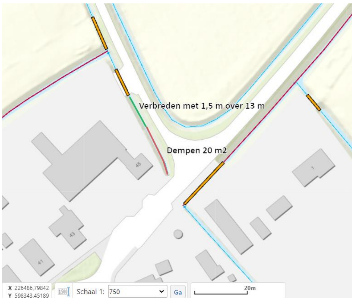
Figuur 1: Schematische tekening van de werkzaamheden. De rode lijn geeft globaal de locatie weer van het te dempen gedeelte van de watergang, de groene lijn geeft globaal de locatie weer van het te verbreden gedeelte van de watergang.
