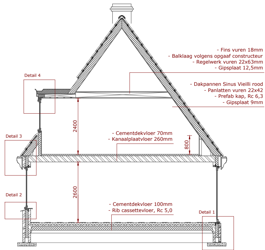
Doorsnede A-A
