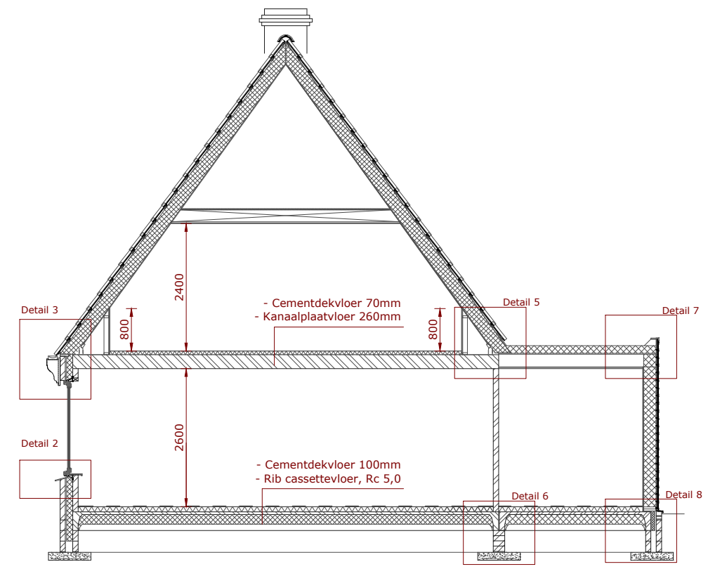
Doorsnede B-B
