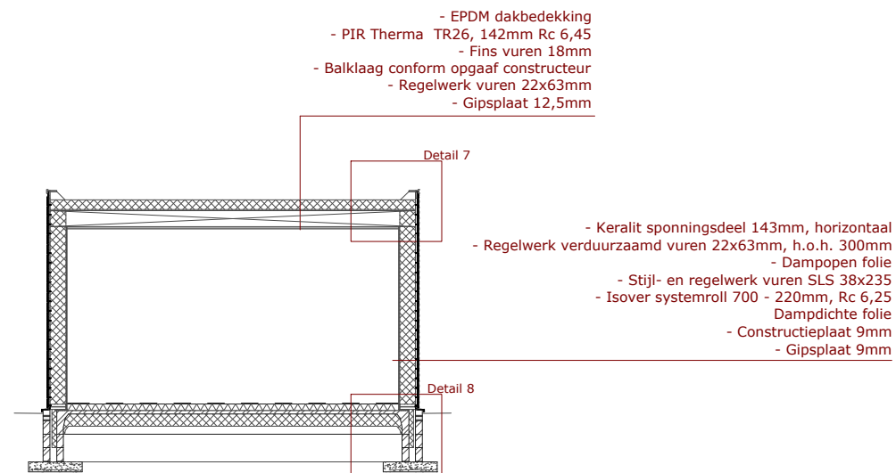
Doorsnede C-C
