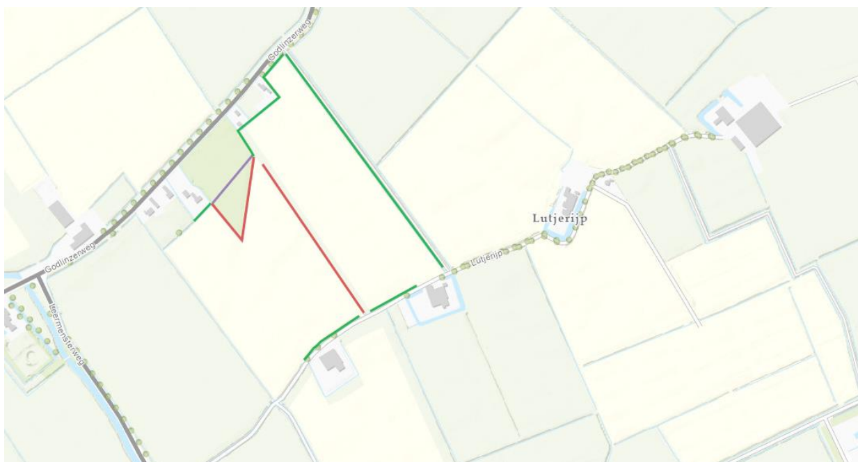
Figuur 1: Locatie van activiteiten. De rode lijnen geven te dempen watergangen weer. De groene lijnen geven te verbreden watergangen weer. De paarse lijn geeft nieuw te graven watergang weer.
