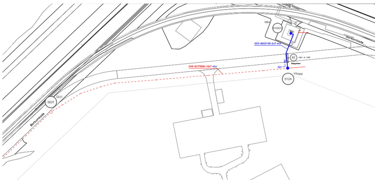
Figuur 1: In het blauw het te graven glasvezelkabeltracé.
