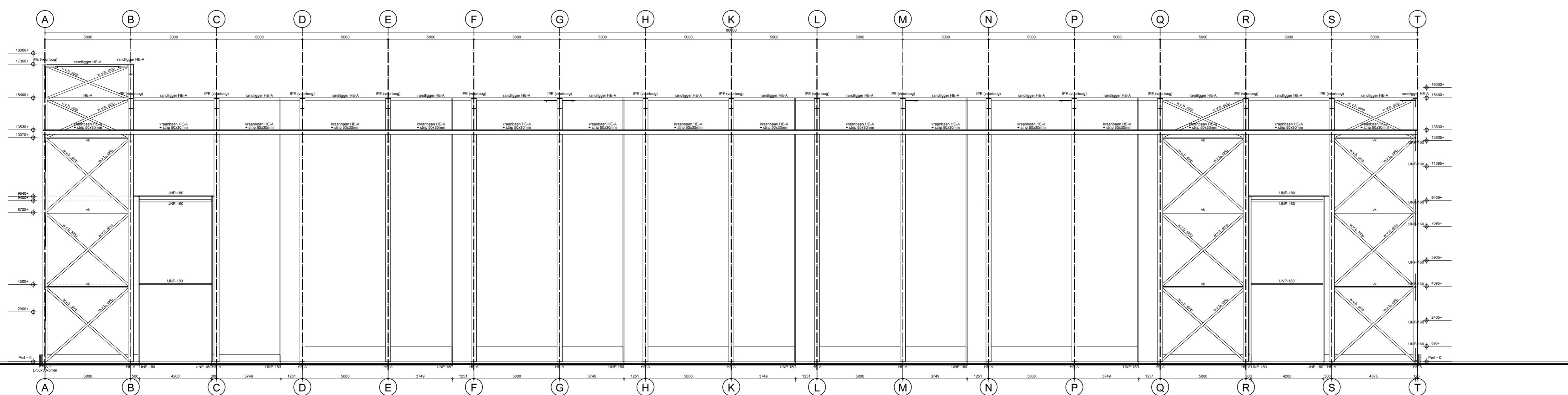
STRAMIEN 07
