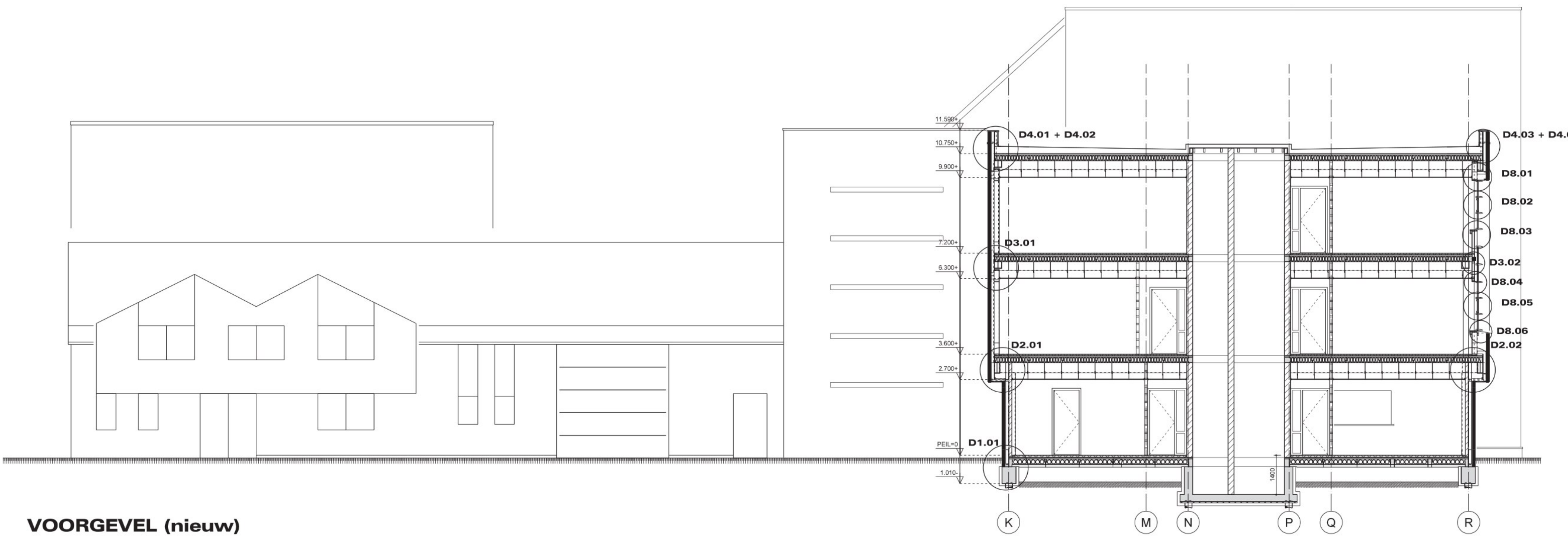
DOORSNEDE A-A
