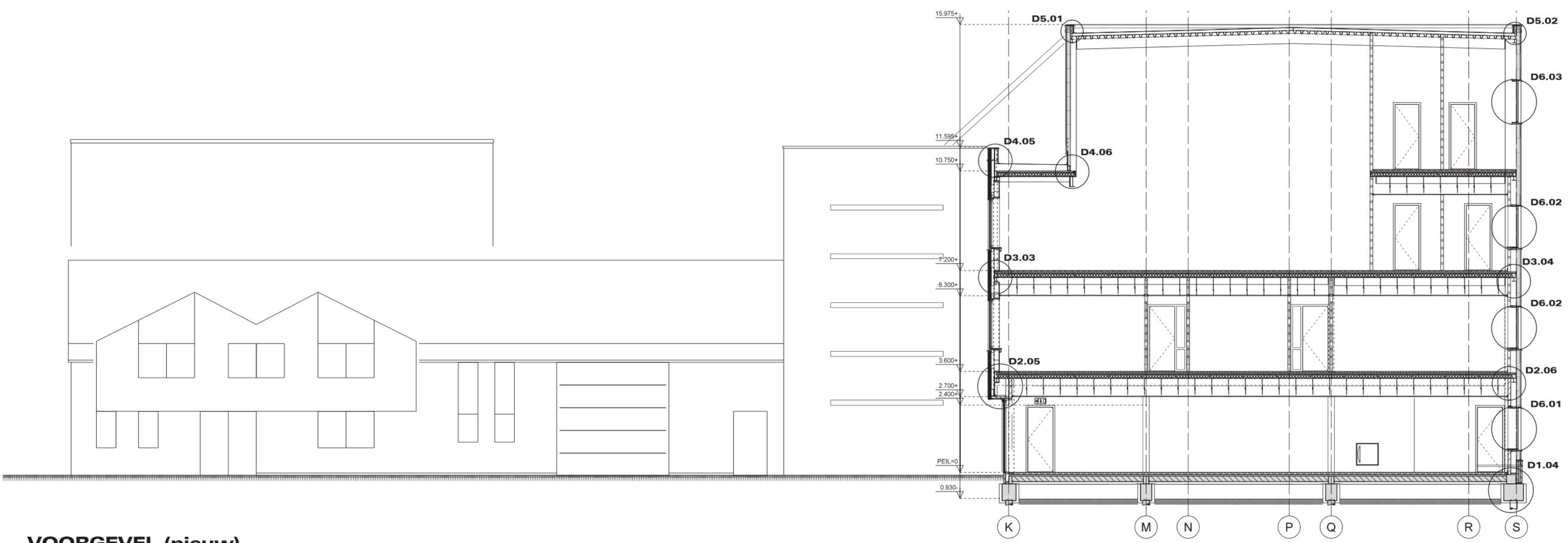
DOORSNEDE C-C
