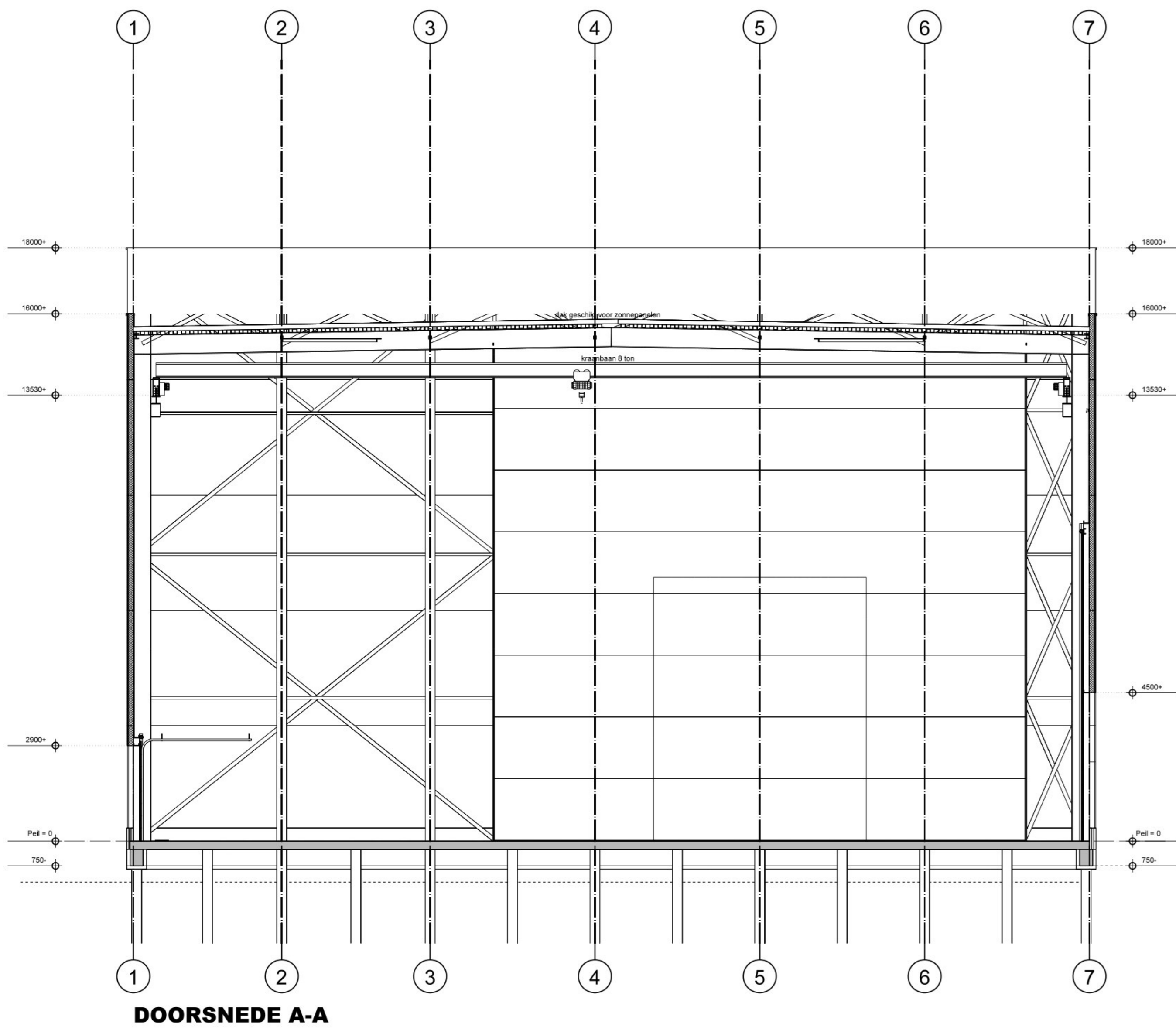
DOORSNEDE A-A
