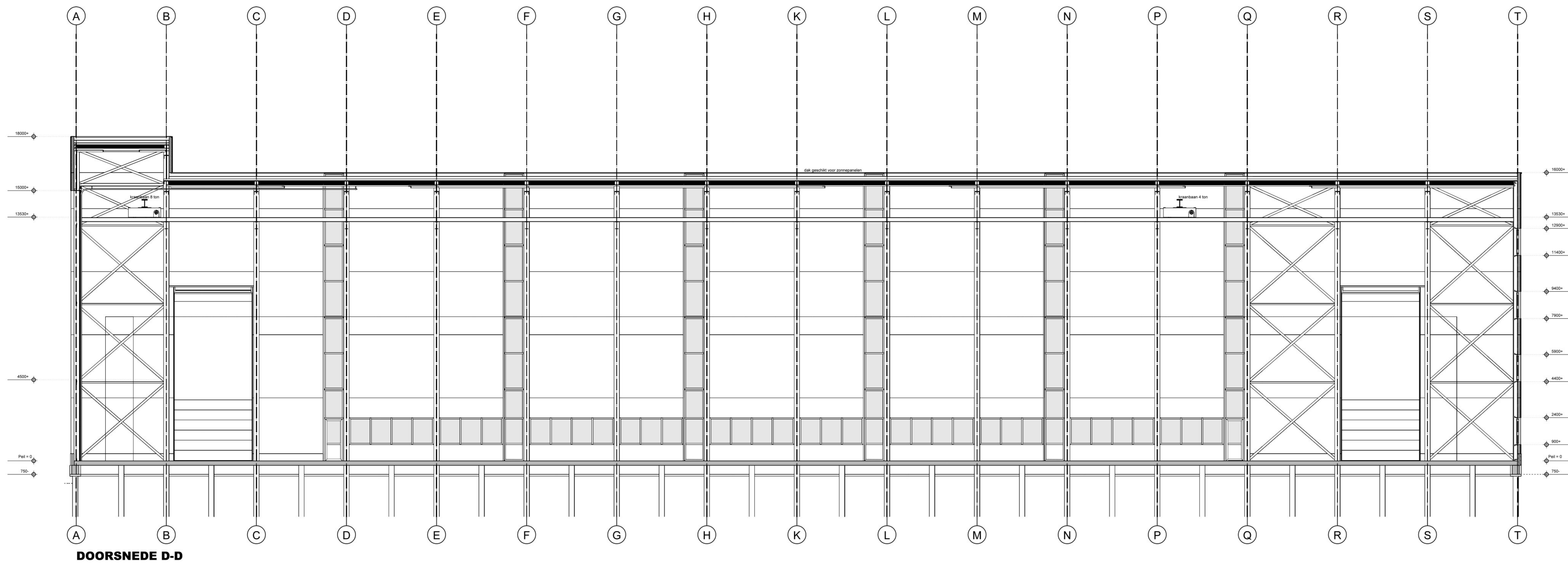
DOORSNEDE D-D
