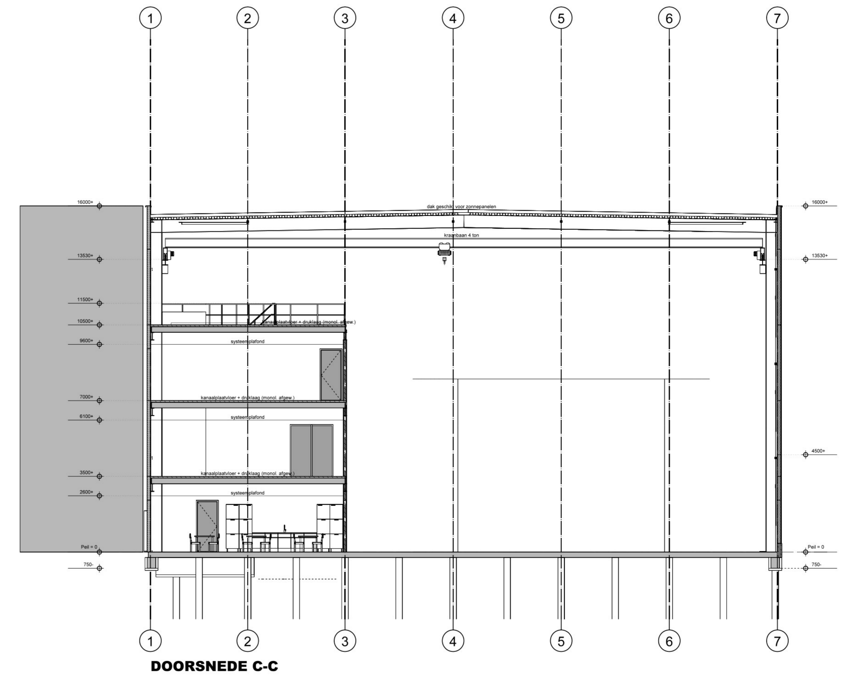
DOORSNEDE C-C
