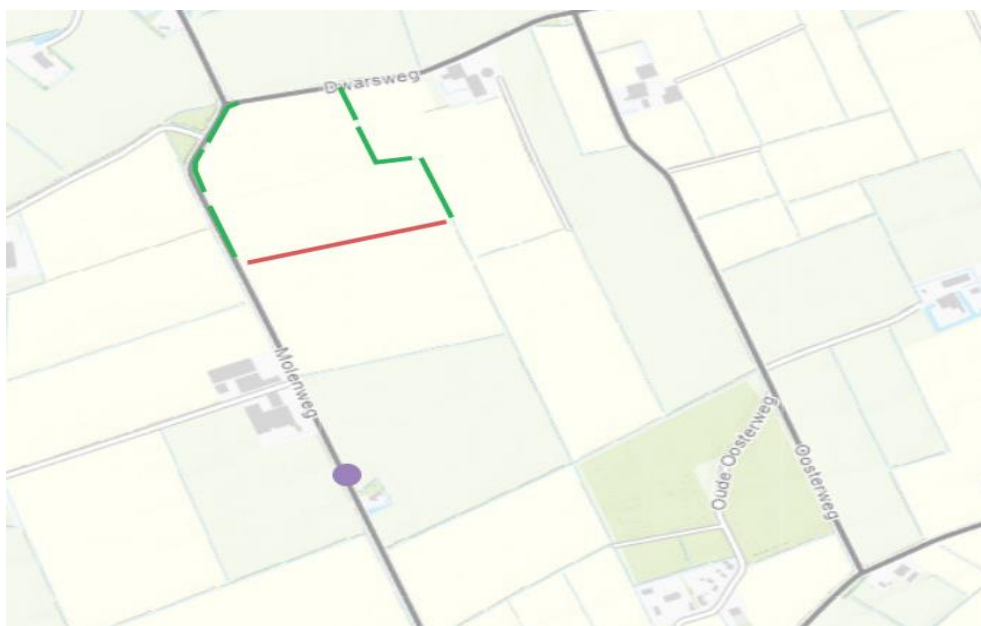
Figuur 1: Locatie van werkzaamheden. De rode lijn geeft de te dempen watergang weer. De groene lijnen geven te verbreden watergangen weer. De paarse stip geeft de locatie van de aan te leggen dam met duiker weer.
