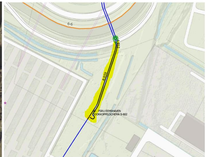
Figuur 2: Detailtekening (geel = locatie)
