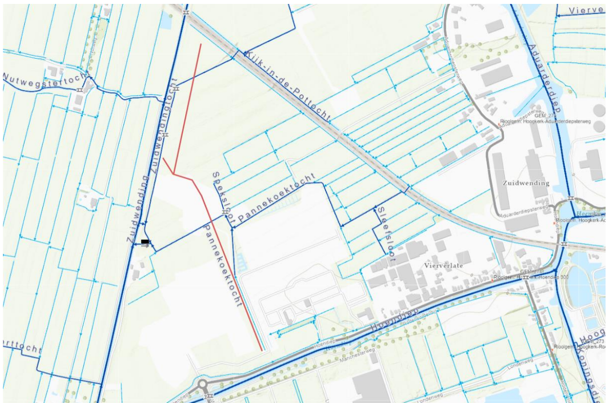
Figuur 1: Schematische tekening van de werkzaamheden. De rode lijn geeft globaal het aan te leggen tracé weer.
