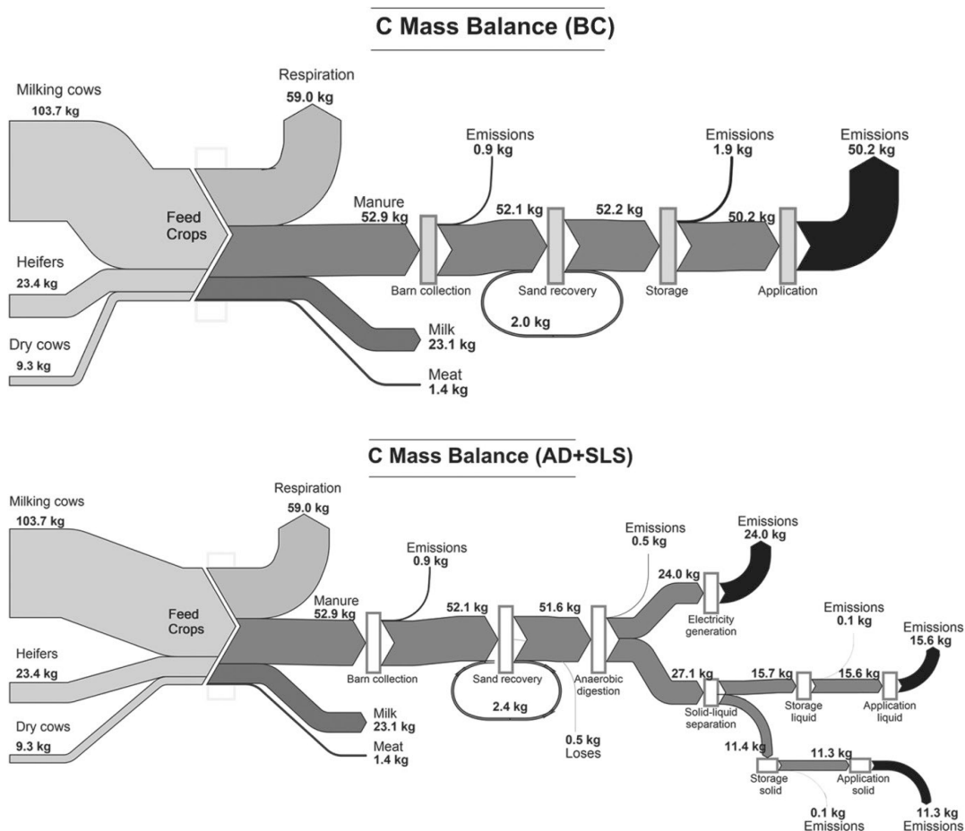
Figuur 2 C massa balans van zonder (boven) en met vergisting inclusief scheiden van digestaat(onder). (AguirreVillegas, 2014). De balans is gebaseerd op 1 ton drijfmest.
