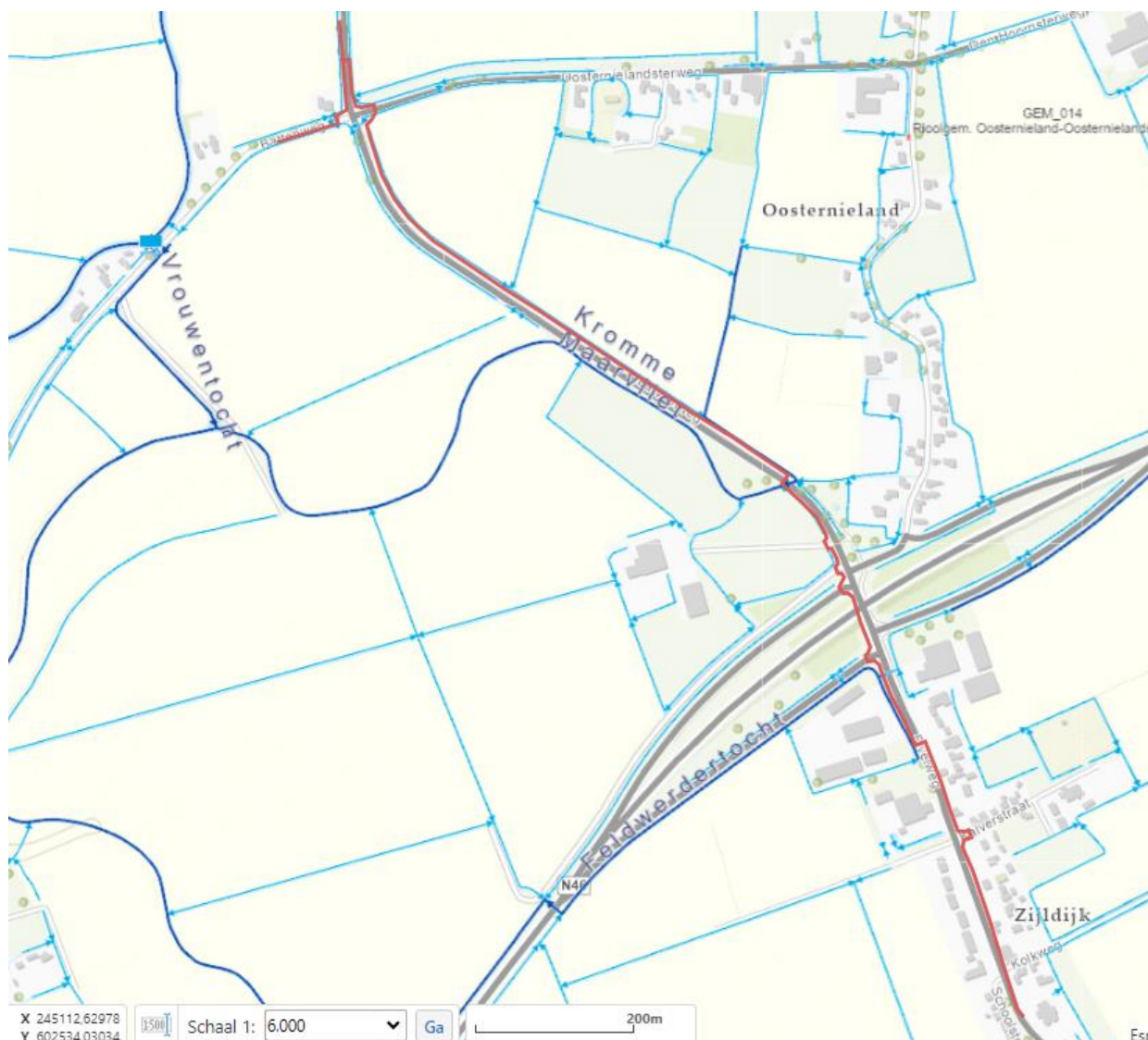
Figuur 1: Schematische tekening van de werkzaamheden. De rode lijn geeft globaal de locatie weer van de het aan te leggen tracé.
