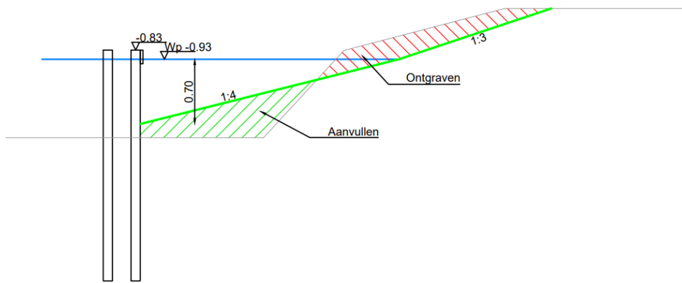
Principeddoorsnede oever Schaal: 1:50
