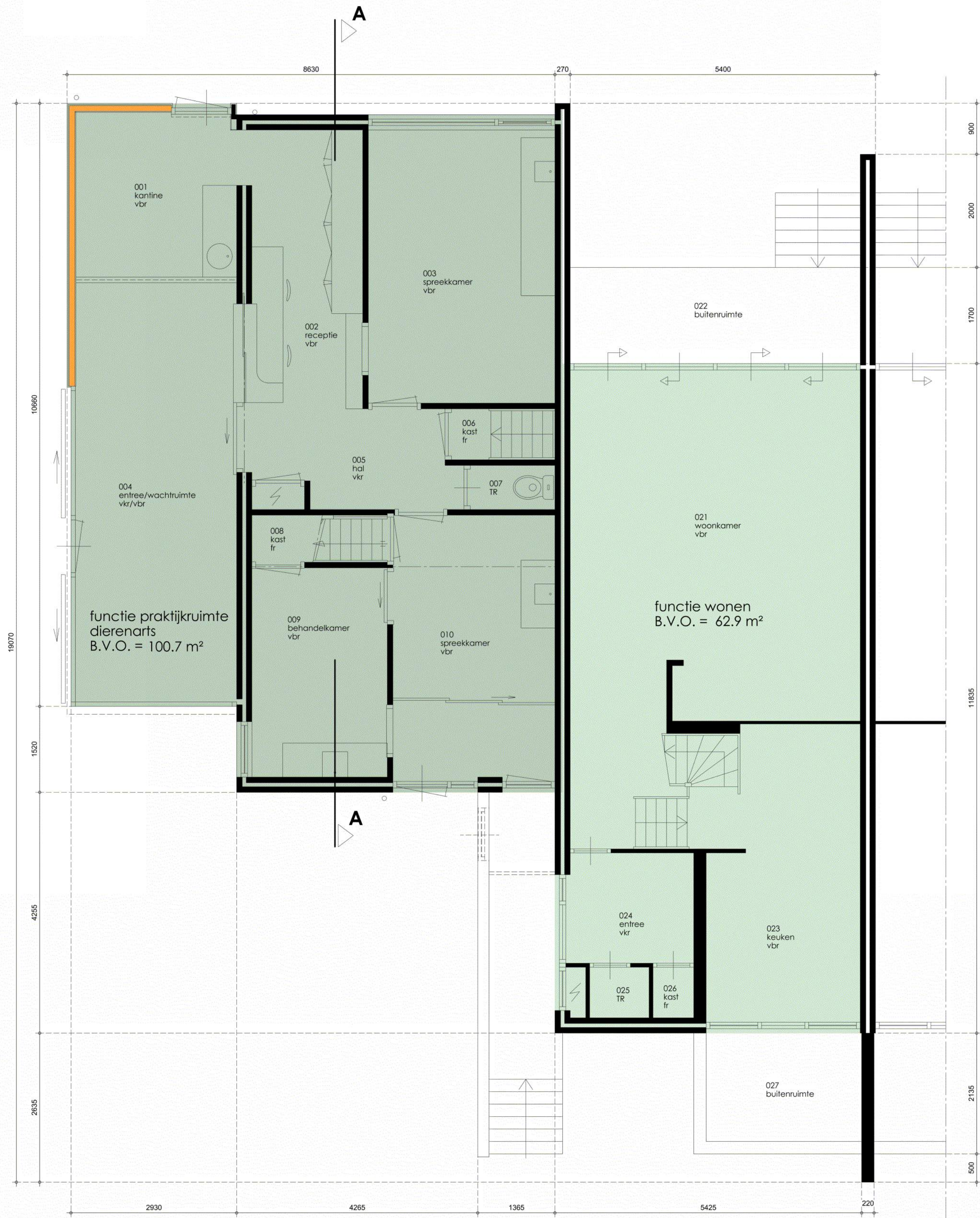
BEGANE GROND bestaande toestand
