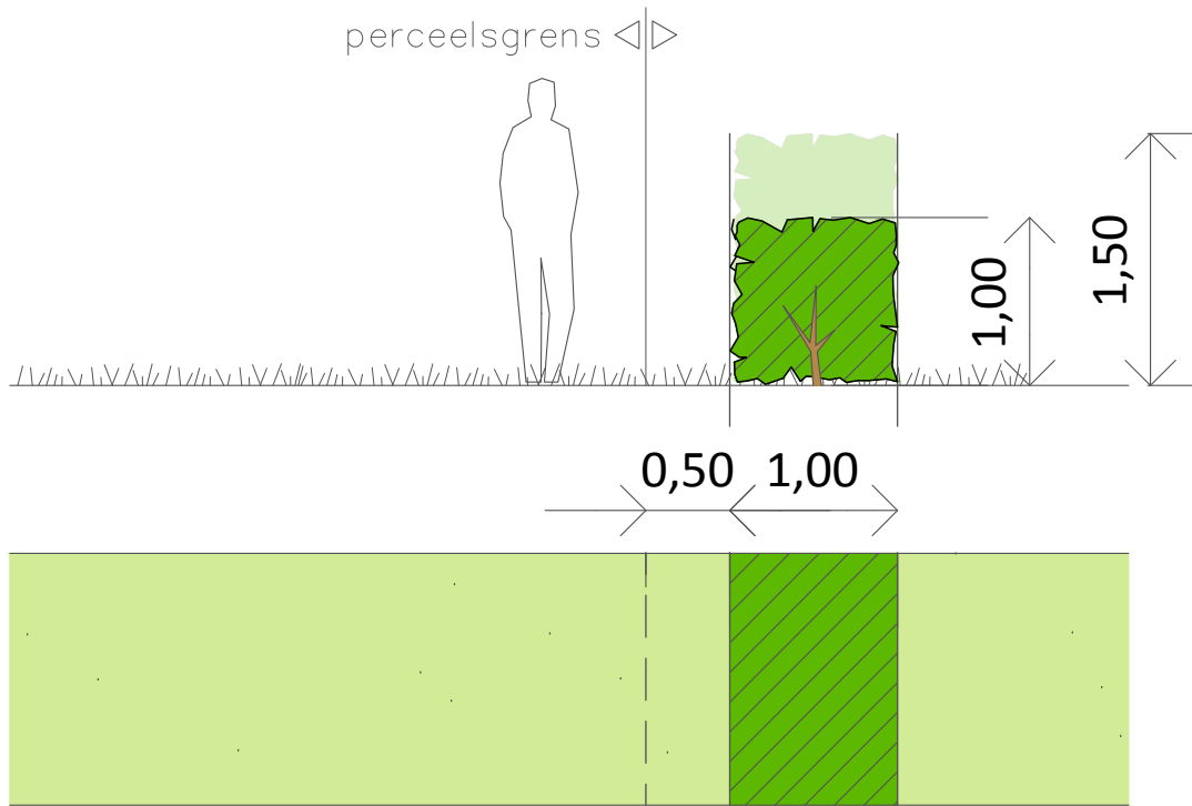
PRINCIPEPROFIEL PLAATSING HAGEN Schaal: 1:50
