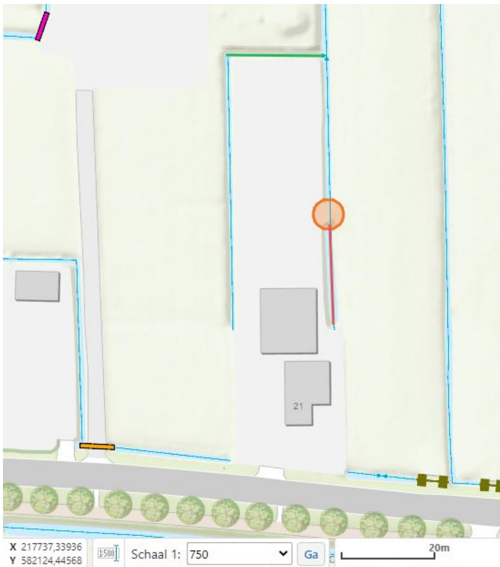
Figuur 1: Schematische tekening van de werkzaamheden. De rode lijn geeft globaal de locatie weer van de te dempen watergang en de oranje cirkel de te verwijderen dam. De groene lijn geeft globaal de locatie weer van de te verbreden watergang.
