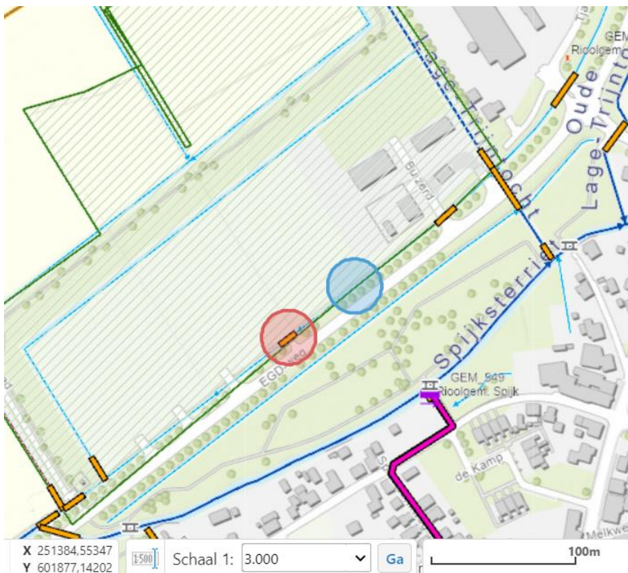
Figuur 1: Schematische tekening van de werkzaamheden. De rode cirkel geeft globaal de locatie weer van de te verbreden dam met duiker. De blauwe cirkel geeft globaal de locatie weer van de nieuw aan te leggen dam met duiker.
