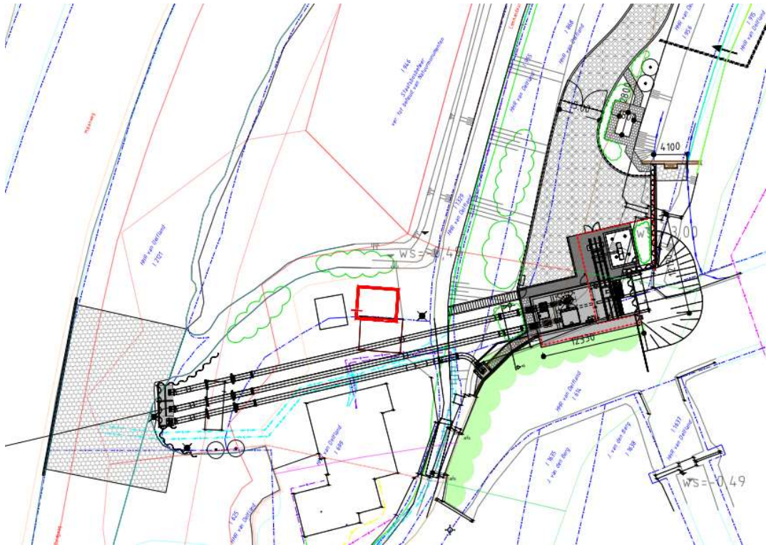
Nieuwe gemaal inclusief ondergrondse leidingen en nieuwe locatie bakhuisje
