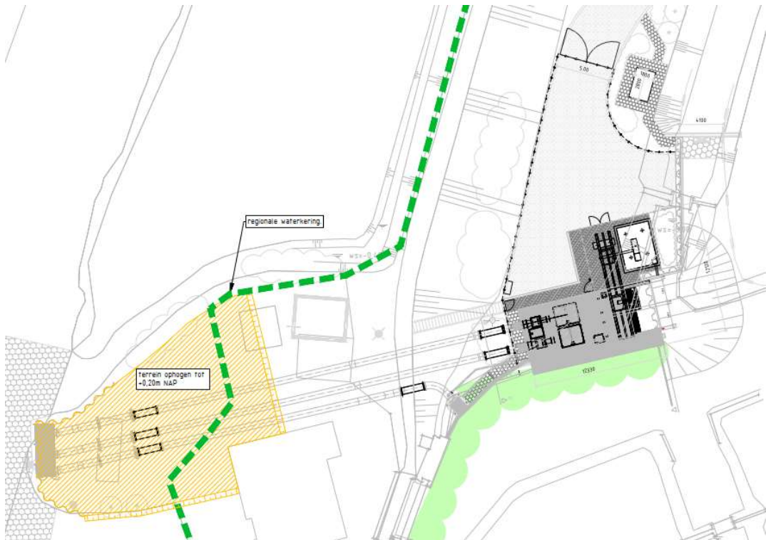
Bovenaanzicht gemaal tekeningnr. 2021-2576 inclusief regionale waterkering
