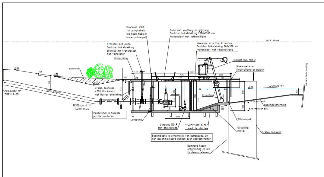
Kragten, technische doorsnede gemaal, uitsnede uit tekeningnr. 2021-1866
