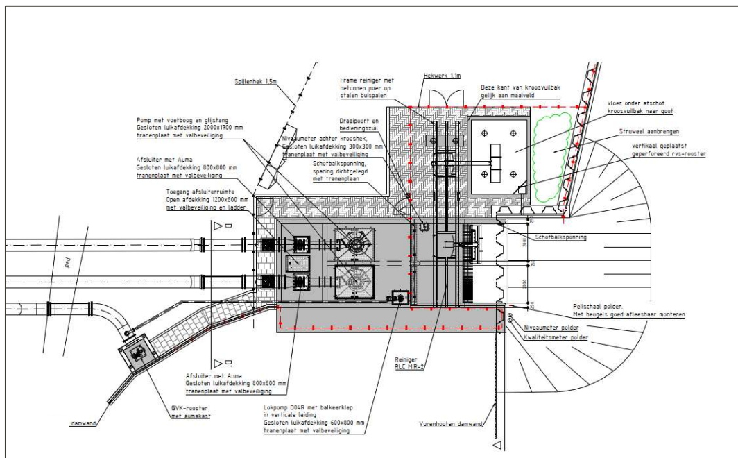
Kragten, technisch bovenaanzicht gemaal, uitsnede uit tekeningnr. 2021-1866
