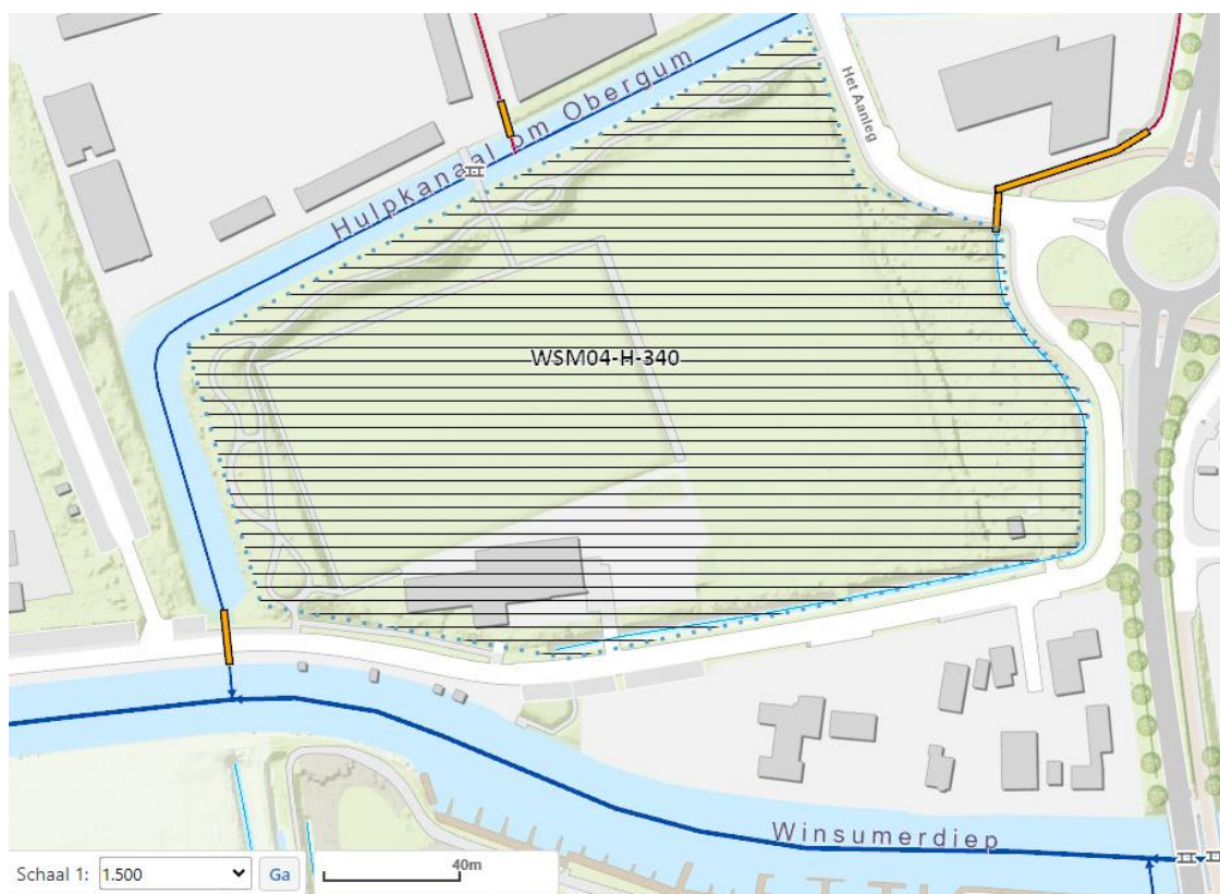
Figuur 1: Tekening overzicht projectlocatie (gestreept kader) van diverse waterhuishoudkundige werkzaamheden ten behoeve van Het Aanleg
