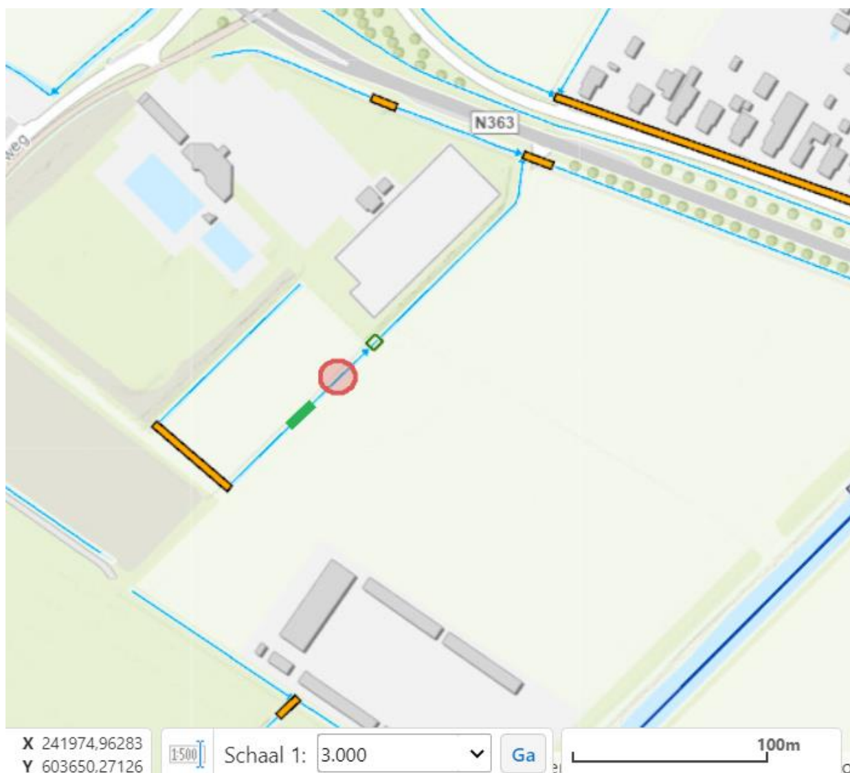
Figuur 1: Schematische tekening van de werkzaamheden. De rode cirkel geeft globaal de locatie weer van de aan te leggen dam met duiker. De groene lijn geeft globaal de locatie weer van het verbreden van de watergang ter compensatie van de verloren waterbergingscapaciteit.
