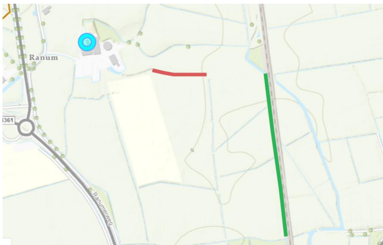
Figuur 1: Locatie van werkzaamheden. De rode lijn geeft te dempen watergang weer. De groene lijn geeft te verbreden watergang middels natuurvriendelijke oever weer.
