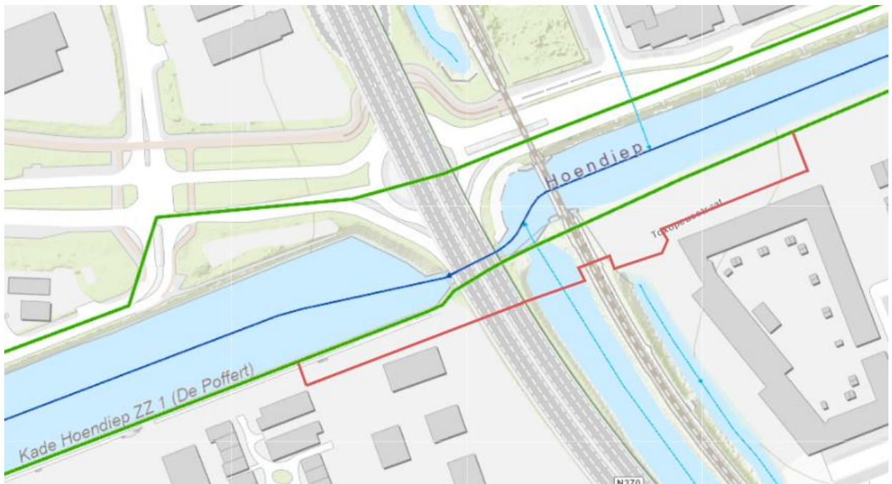
Bijlage 2: Tekening met in het rood globaal het nieuwe waterkeringstracé (groen = het bestaande tracé)
