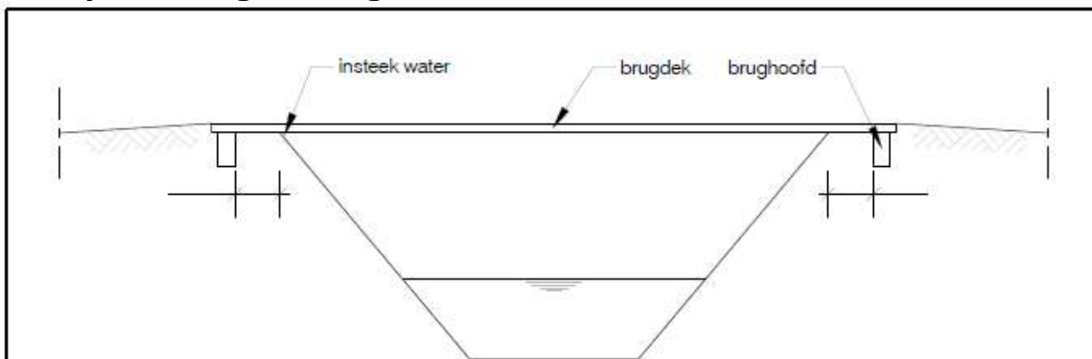
Dwarsdoorsnede A-A
