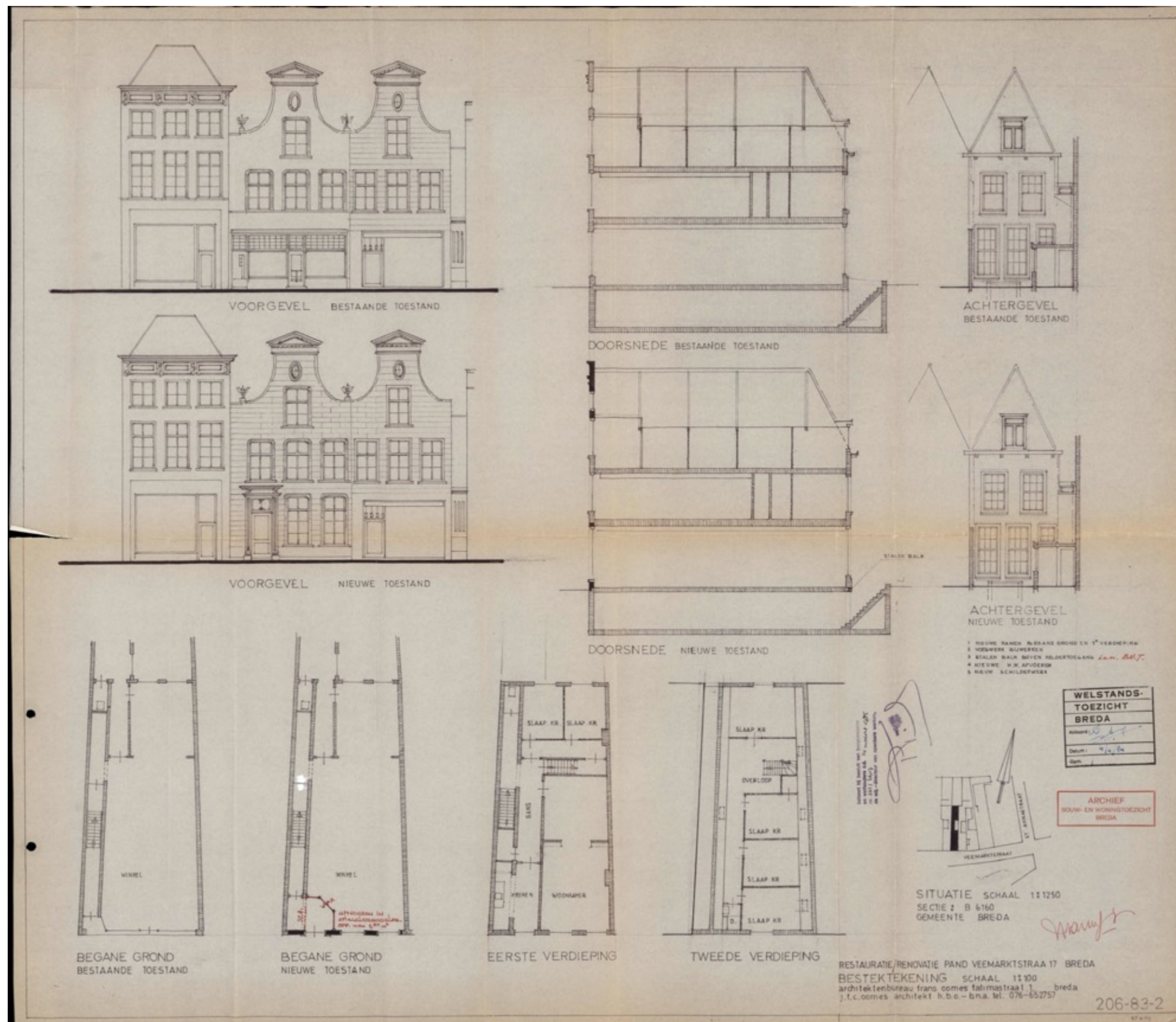
Afb. 77: Bouwtekening uit 1985. [Stadsarchief Breda]
