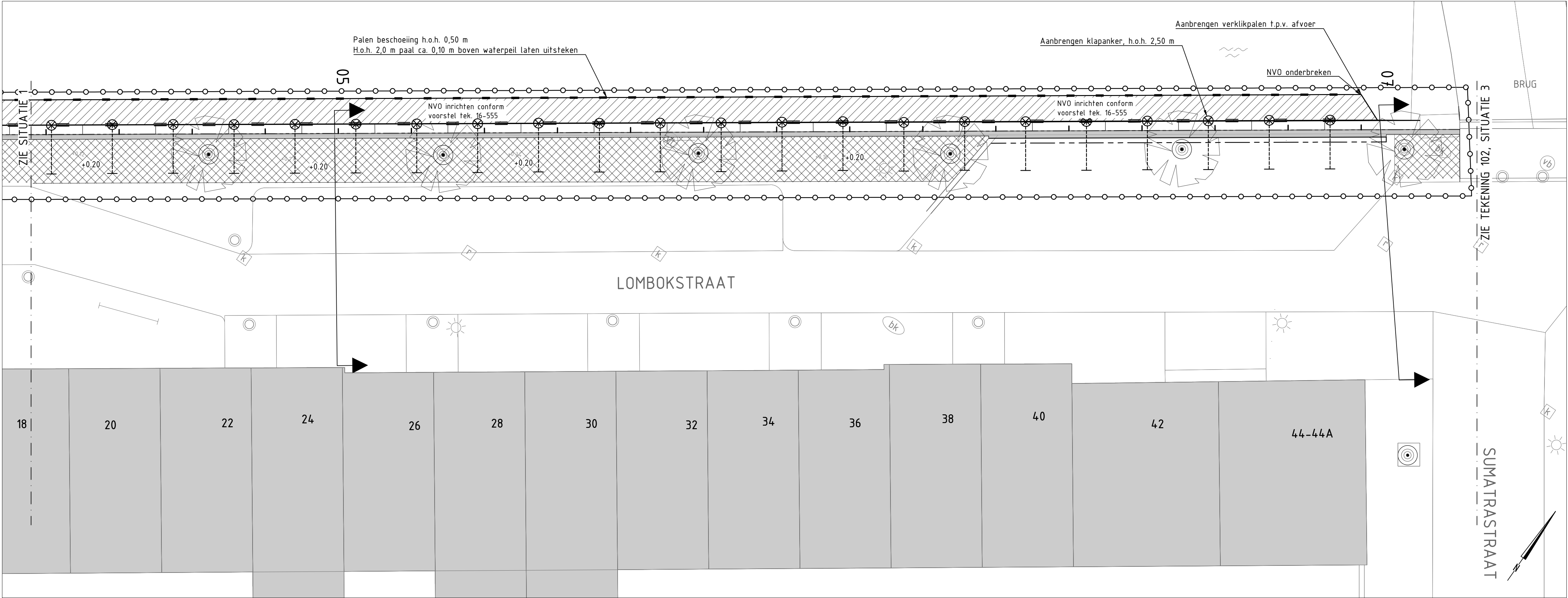
SITUATIE 2 Schaal 1:100
