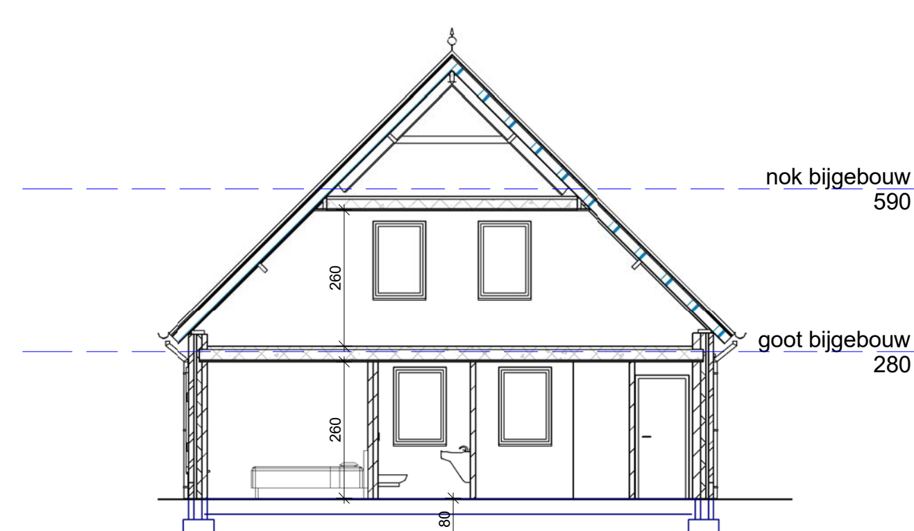
Doorsnede B
