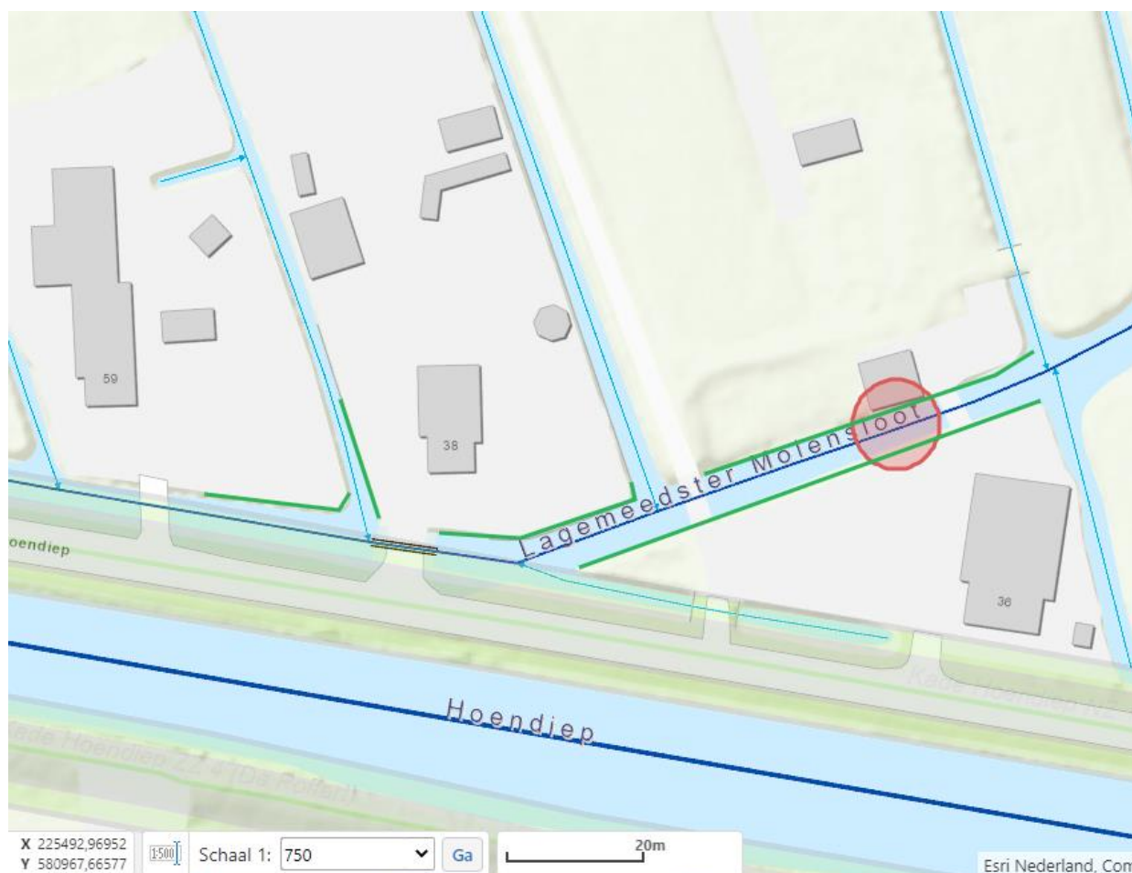
Figuur 1: Schematische tekening van de werkzaamheden. De rode cirkel geeft globaal de locatie weer van het verwijderen van de bestaande brug en de aan te leggen dam met duiker, de groene lijnen geven de aan te leggen beschoeiing weer.
