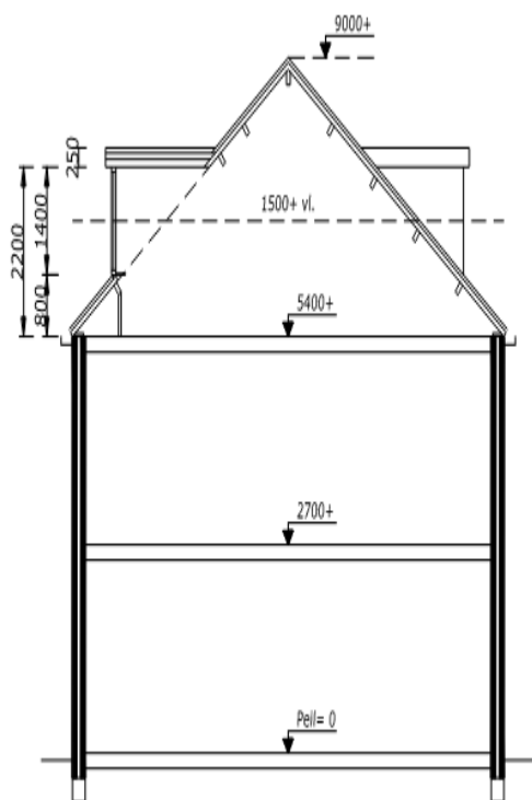
DOORSNEDE GEWIJZIGD
